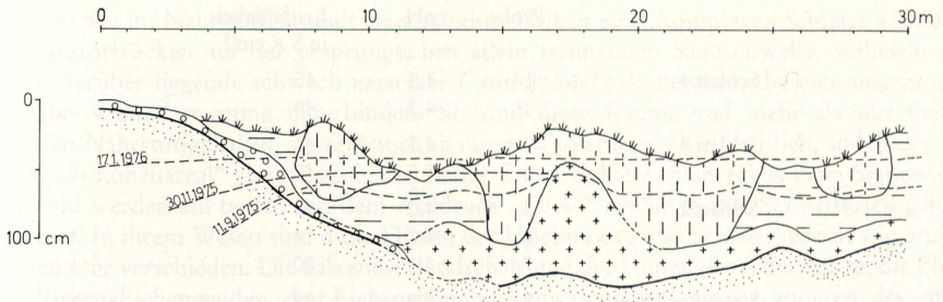
Abb.7: Schnitt durch Schlatt 8 in den Osenbergen mit Wasserständen zu verschiedenen Zeitpunkten
