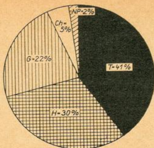
Abb. 7. Lebensform-Spektrum der Flora von Scharhörn.
