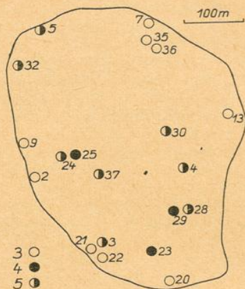
Abb. 3. Lage der Aufnahmen: 3 des Elymo-Agrophyretum juncei (Tab. 3), 4 der Agropyron littorale -Ges. (Tab. 4) und 5 des Elymo-Ammono-philetum (Tab. 5) auf Scharhörn.
