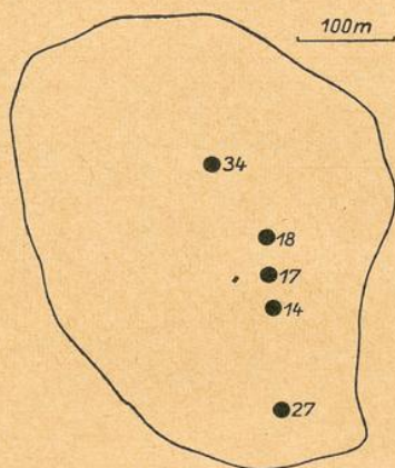
Abb. 6. Lage der Aufnahmen des Koelerion albescentis auf Scharhörn (Tab. 6).
