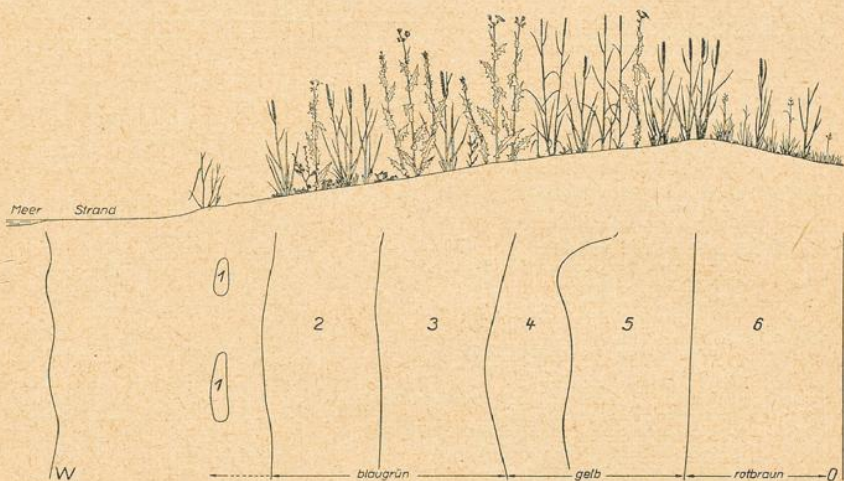
Abb. 5. Schematische Gesellschafts-Zonierung auf der w Randdüne von Scharhörn (Schnitt und Karte):
