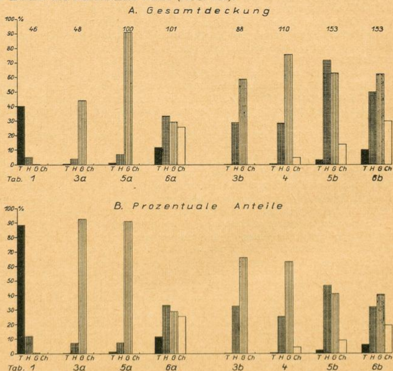
Abb. 8. Lebensform-Spektren der Pflanzengesellschaften von Scharhörn.
