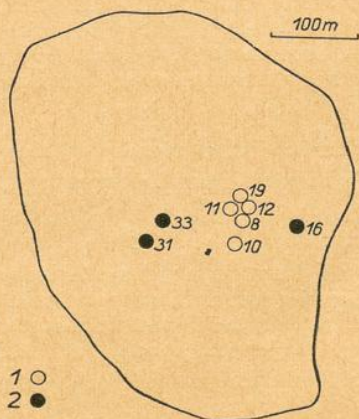
Abb. 1. Lage der Aufnahmen: 1 des Atriplicetum littoralis chenopodietosum (Tab. 1) u. 2 der Agrostis stolonifera - Potentilla anserina -Ges. (Tab. 2) auf Scharhörn.
