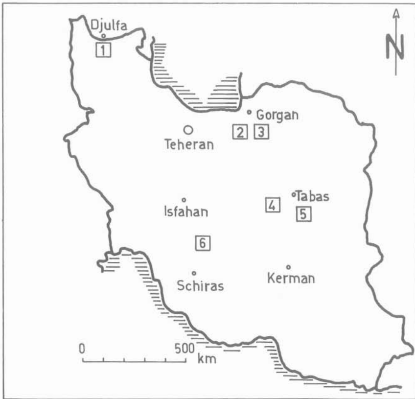
Abb. 1: Lage-Übersicht der behandelten Korallen-Fundpunkte des Iran (siehe auch K. METZ 1961, W. GRÄF 1964).
