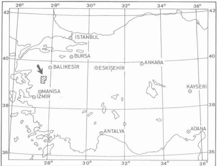
Abb. 1: Geographische Lage des Braunkohlengebietes von Soma in Westanatolien.
