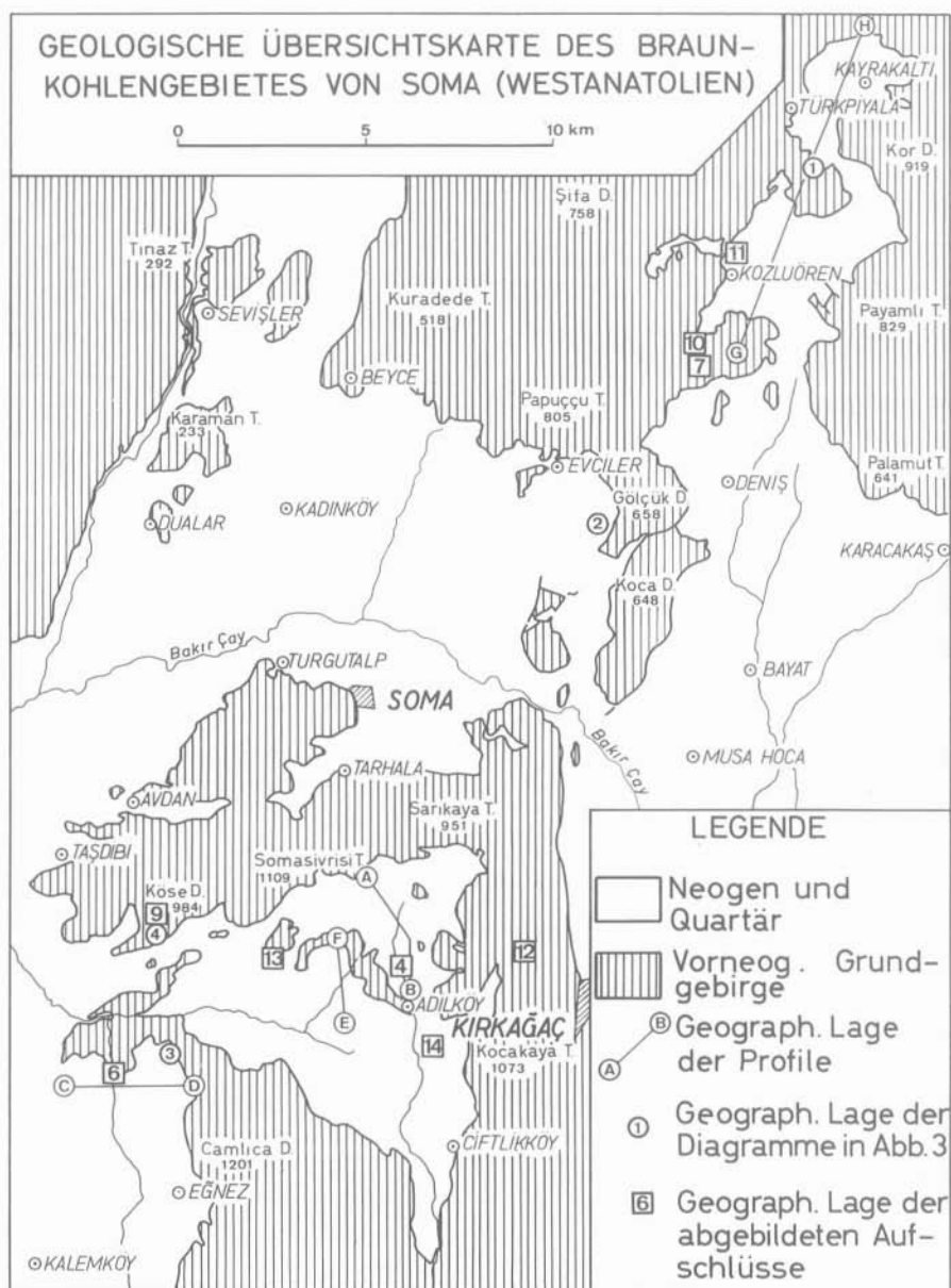
Abb. 2: Geologische Übersichtskarte des Braunkohlengebietes von Soma (Westanatolien).
