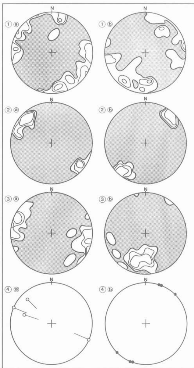
Abb. 3: Strukturdiagramme von Harnischstreifen (a) und Harnischflächenpolen (b). Die geographische Lage der dazugehörigen Aufschlüsse ist Abb. 2 zu entnehmen. Anzahl der eingemessenen Harnischstreifen: Diagr. 1 a = 30; Diagr. 2 a = 13; Diagr. 3 a = 34; Diagr. 4 a = 3. Anzahl der eingemessenen Harnischflächen: Diagr. 1 b = 30; Diagr. 2 b = 13; Diagr. 3 b = 23; Diagr. 4 b = 3. Besetzungsdichte bei den Diagrammen mit Begrenzungslinien: 1 %, 5 % und 10 %.
