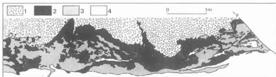
Abb. 11: Zerschnittenes Lignit-Glied ( k_1 ) in einem Schurfstollen. 1 = tektonische Brekzie; 2 = Kohlenstaub; 3 = mit Kohle vermengter Ton; 4 = m_2 -Mergel. (Geograph. Lage des Aufschlusses s. Abb. 2.) Nach einer Fotografie gezeichnet.
