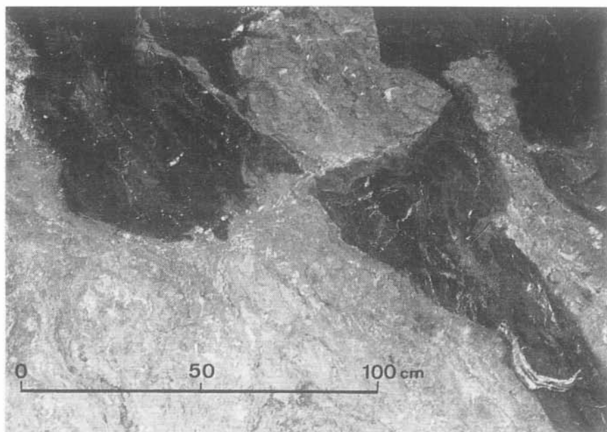
Abb. 12: Tektonische Melange, bestehend aus Kohlenrümern des unteren Lignit-Gliedes ( k_1 ) und den zu einer tektonischen Brekzie umgewandelten m_2 -Mergeln. Der Aufschluß liegt etwa 1 km nördlich der Ortschaft Kozluören (s. Abb. 2).
