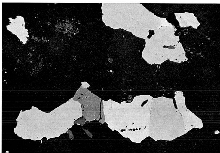
Abb. 2: Vererzung Lehnermühle. Magnetkies (lichtgrau, durch Reflexionspleochroismus verschiedene Töne) ist mit Zinkblende (mittelgrau, links unterhalb Bildmitte) und kleinen Graphitaggregaten (licht- bis dunkelgrau, Reflexionspleochroismus!) sowie mit etwas Kupferkies (Spur heller als Magnetkies, rechte obere Bildhälfte) verwachsen. Kupferkies dringt entlang Korngrenzen in Magnetkiesverwachsungen ein. Die Zinkblende zeigt schwache Magnetkiesentmischung. Randlich am Magnetkies findet sich etwas Titanit (dunkelgrau), in der Gangart Graphit (besonders linke obere Bildhälfte). Anschliff, Vergr.: 85×.
