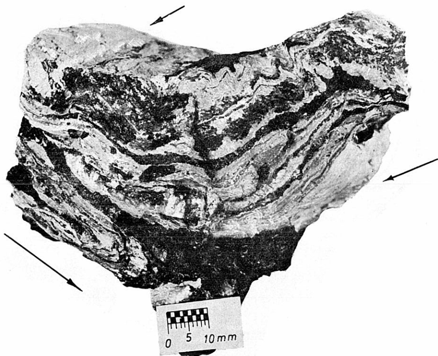
Abb. 2: Rabenstein. Gleiche Probe wie in Abb. 1, Rückseite. Deutlich ist eine dis-harmonische Faltung bzw. Fältelung und ein unterschiedliches Ausdünnen und Verdicken der konkordanten Erzlagen (schwarz) mit Einpressung in Faltenkerne zu beobachten. Auftretende Faltenachsen (stark divergierende Achsenrichtungen!) wurden, sofern in der Abbildung noch erkennbar, durch Pfeile dargestellt. Wie in Abb. 1 finden sich Anflüge von sekundärem Pyrit (dunkel-grau bis schwarz).
