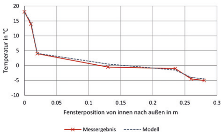
BILD 3. TEMPERATURPROFIL ÜBER DIE TIEFE DER KASTENFENSTERKONSTRUKTION MIT ÜBERLAGERTEM MODELL [6]
