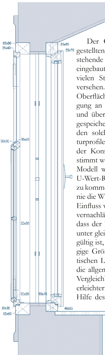
BILD 2. SCHNITTDARSTELLUNG DER BETRACHTETEN DOPPELFENSTER-KONSTRUKTION [6]
