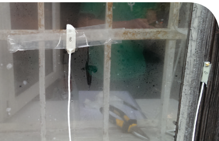
BILD 1. BETRACHTETE DOPPELFENSTERKONSTRUKTION AM BENEFIZIUM HALLSTATT.
