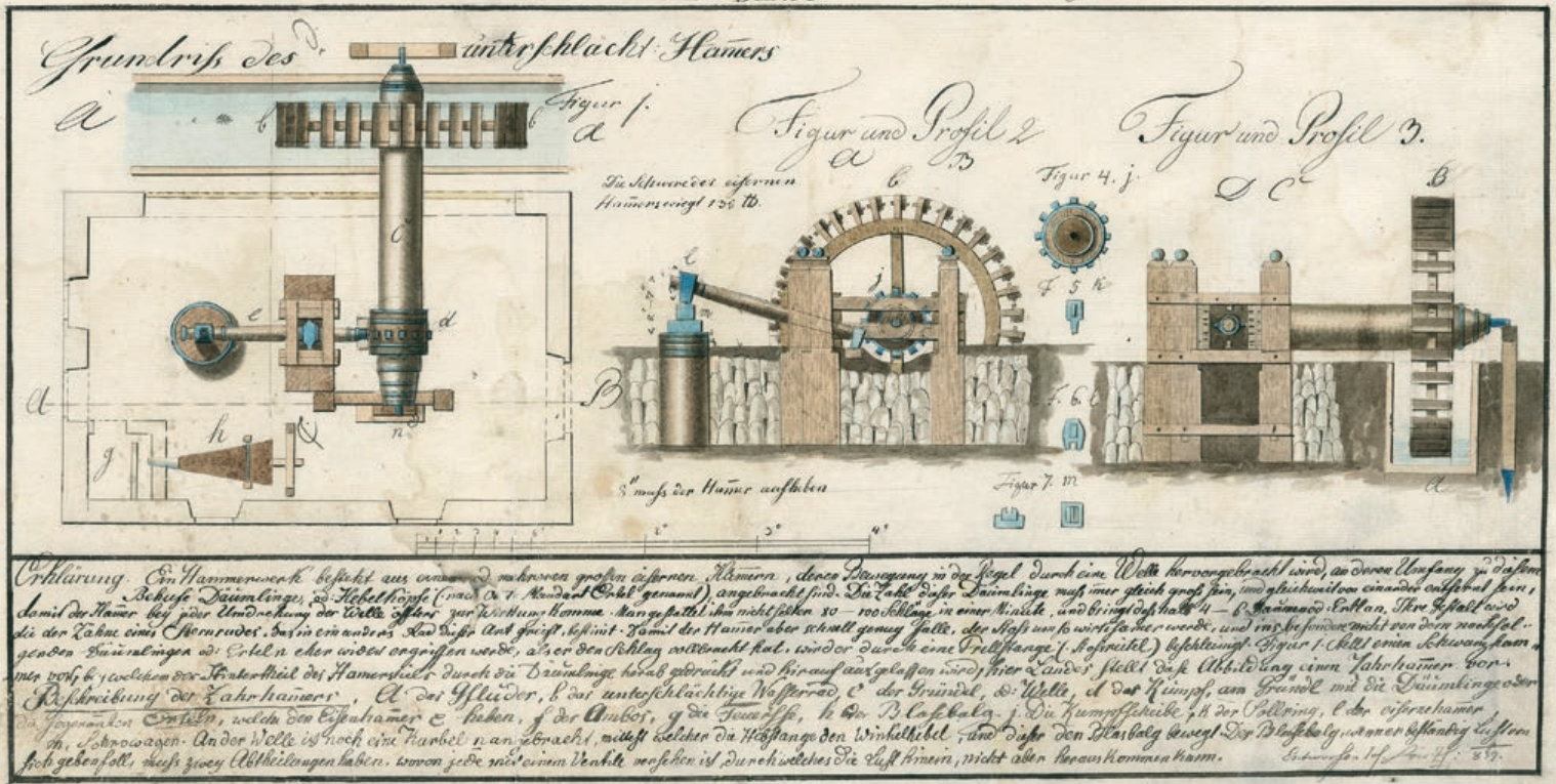
DAS JÜNGST RESTAURIERTE BLATT XV EINES UMFANGREICHEN ZYKLUS TECHNISCHER ZEICHNUNGEN VON JOSEPH LÖW, ANGEFERTIGT FÜR CASPAR ZEITLINGER.
