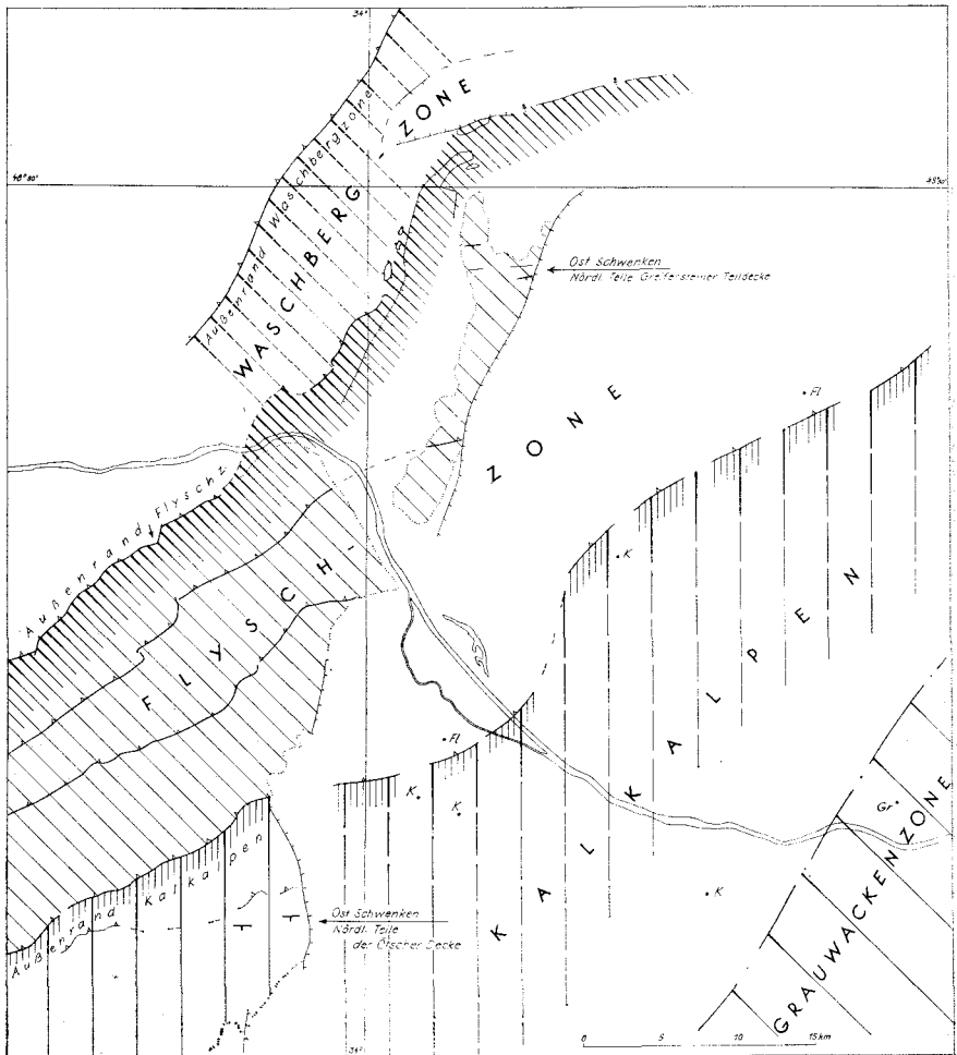
Schematische Skizze der Verknüpfung der tektonischen Einheiten im Grenz- bereich Alpen—Karpaten
