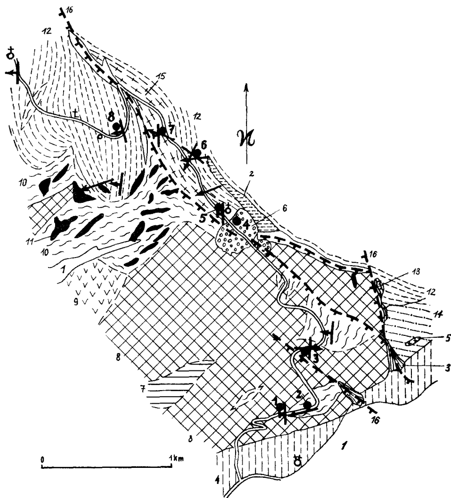
Abb. 7: Geologische Skizze der Gurker Störung
