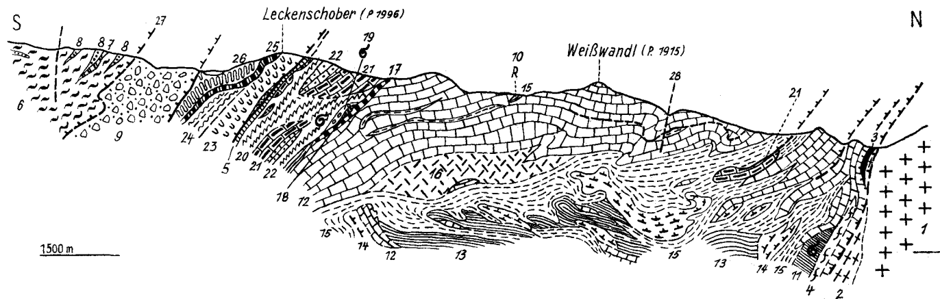
Abb. 6: Leckenschöberprofil Von P. Beck-Mannagetta Unterlagen: H. Stowasser 1956 (A. Tollmann 1958)
