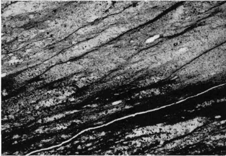
Abb. 13: „Pyritschiefer“, limonitreich, von Breitenstein; völlig anderer Typ der Zerscherung (ss horizontal); ohne Analysator, ca. 30×
