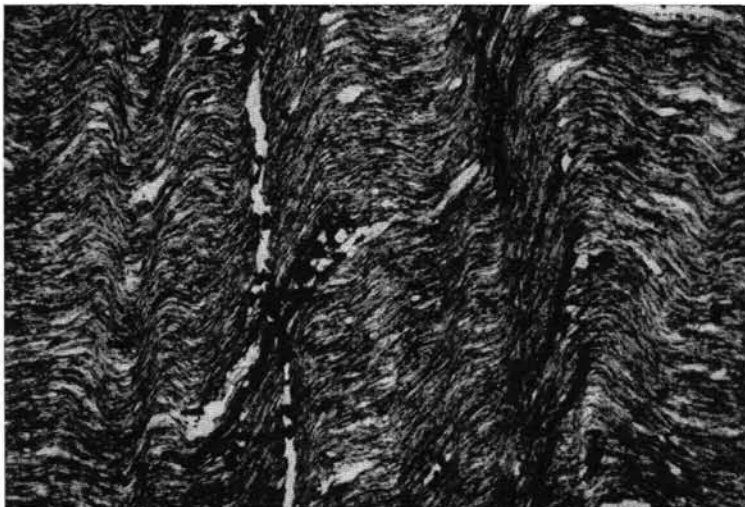
Abb. 6: Graphitphyllit; nach dem gefältelten s_1 dunkle, schnurartig angeordnete, feinkörnige limonitische Aggregate; s_2 vertikal; ohne Analysator, ca. 30\times
