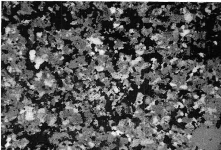
Abb. 10: Limonit- und karbonatreiche, „rostige“ Arkose; schräg gekreuzte Nicols, ca. 30×
