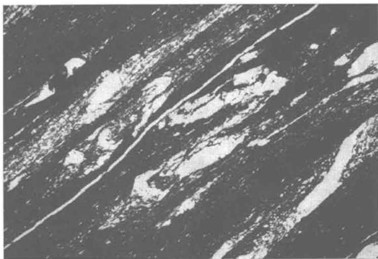
Abb. 4: Graphitphyllit; zerscherte Quarzbänkchen s_1 ; ohne Analysator, ca. 30\times
