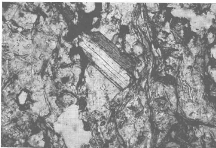
Abb. 8: Sandstein; Hell- und Dunkelglimmer in Parallelverwachsung; ohne Analysator, ca. 190×
