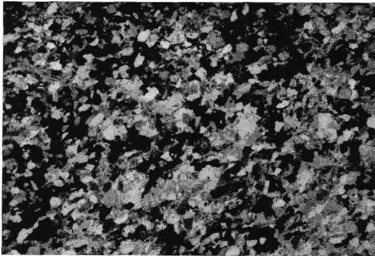
Abb. 14: Limonit- und feldspatreicher Lunzer Sandstein (Feldspäte zersetzt, grau gesprenkelt); schräg gekreuzte Nicols, ca. 30× (vgl. Abb. 10)
