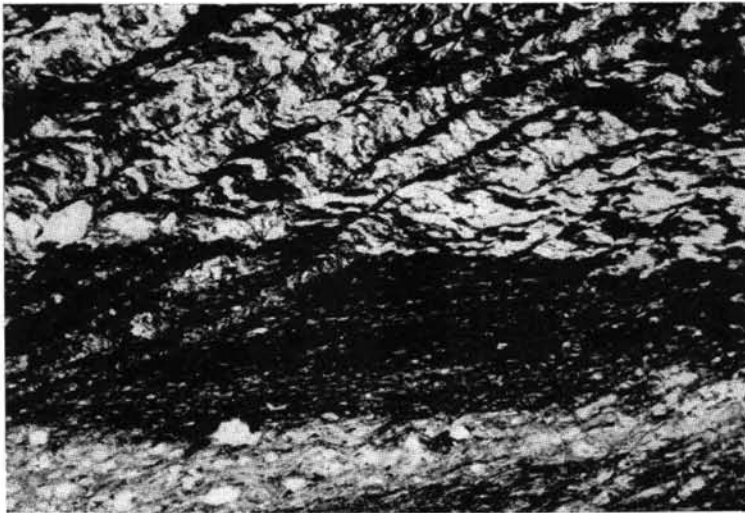
Abb. 5: Graphitphyllit; ss (horizontal), gefältelt s_1 , vom schief dazu liegenden s_2 flexurartig verworfen; ohne Analysator, ca. 30\times
