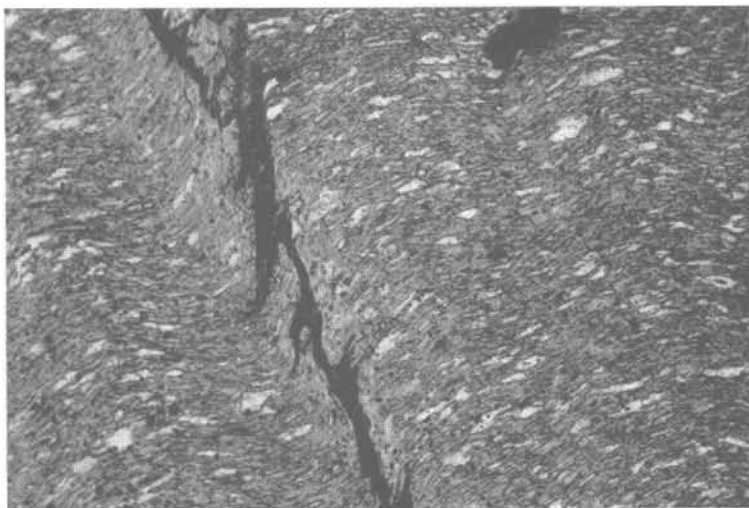
Abb. 3: Graphitfreier Phyllit; Limonit nach s_2 ; ohne Analysator, ca. 75\times
