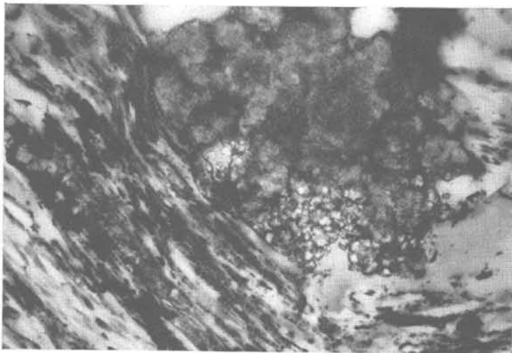
Abb. 7: Graphitphyllit; limonitisches Aggregat; schräg gekreuzte Nicols, ca. 480×
