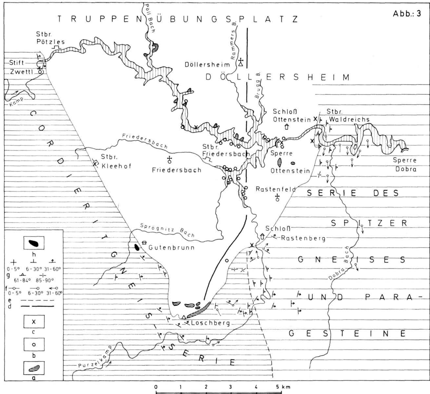
Abb. 3: Kartenskizze der großen Dioritschollen, der Grobkorn-granit- bis Pegmatoidschöte und der Nebengesteinsschollen im Rastenberger Granodiorit sowie der linearen und flächigen Parallelgefüge im Nebengestein des Plutons.
