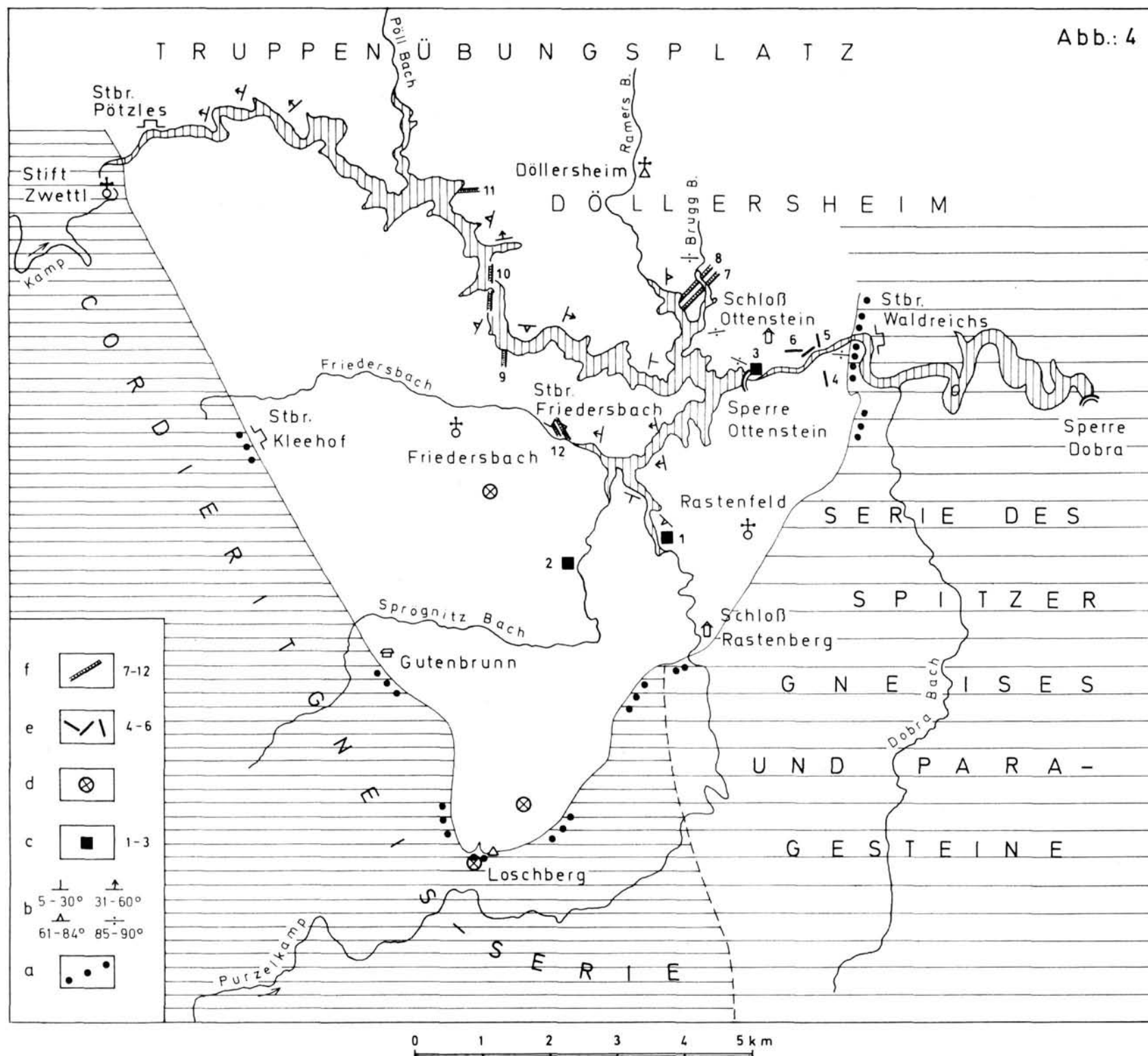
Abb. 4: Kartenskizze einiger ausgewählter Beispiele aus dem Ganggefolge im Rastenberger Pluton.
