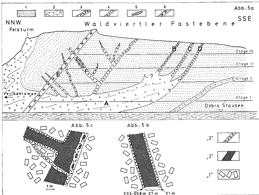
Abb. 5a: Probe-Entnahmestellen einiger Gangtypen im Steinbruch Waldreichs. Es handelt sich bloß um eine beiläufige Skizze und noch nicht um eine genaue geologische Detailaufnahme des Steinbruches. Die Probe-Entnahmestellen „A“ bis „F“ beziehen sich auf die betreffenden Gesteinsbeschreibungen im Text!
