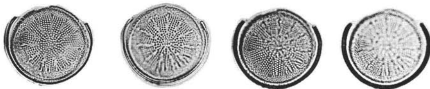
Stephanodiscus kanitzii Pant. Grun. f. minor n. f.
