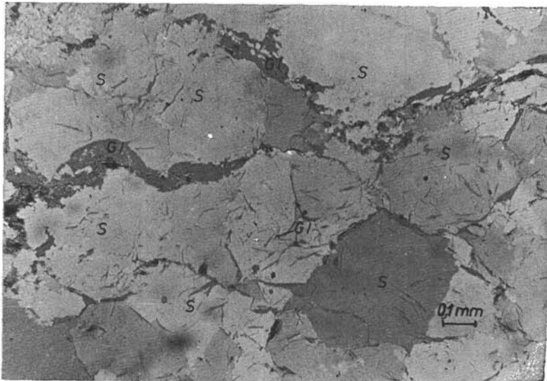
Bild 4: Serizit in Lagen und als Einschluß im Siderit — Anschliff (S = Siderit; Gl = Serizit).
