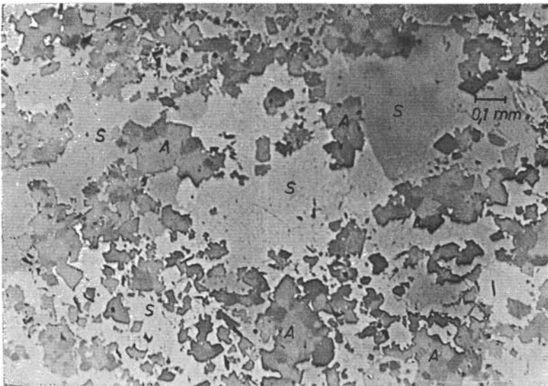
Bild 2: Innige Siderit-Ankerit-Verwachsung — Anschliff (S = Siderit; A = Ankerit, Typus Hangendscholle).
