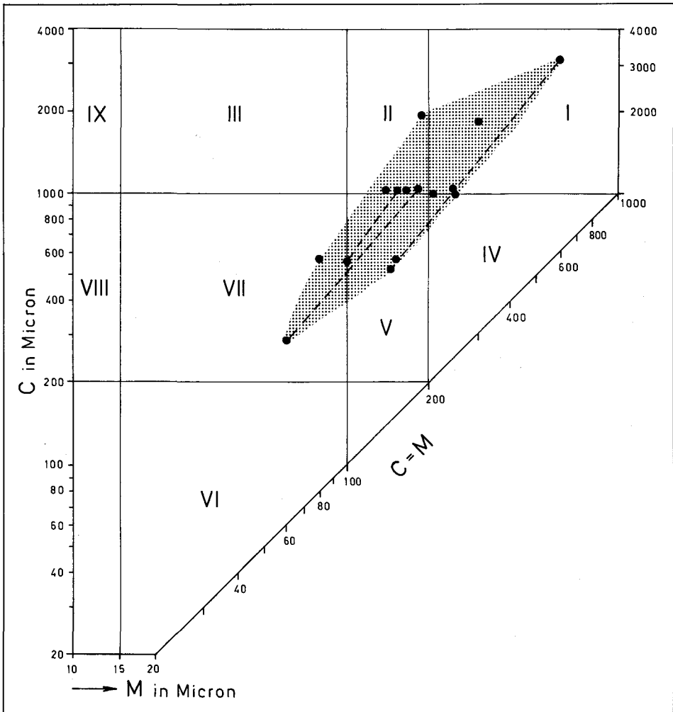
Abb. 10: CM-Diagramm nach PASSEGA mit den Projektionspunkten der Sandsteine der Turbiditätsfazies. M = Median, C = 1%-Perzentil (größter Bereich der Summenkurve). Projektionspunkte des Liegend- und Hangendabschnittes ein und derselben Bank sind miteinander verbunden.
