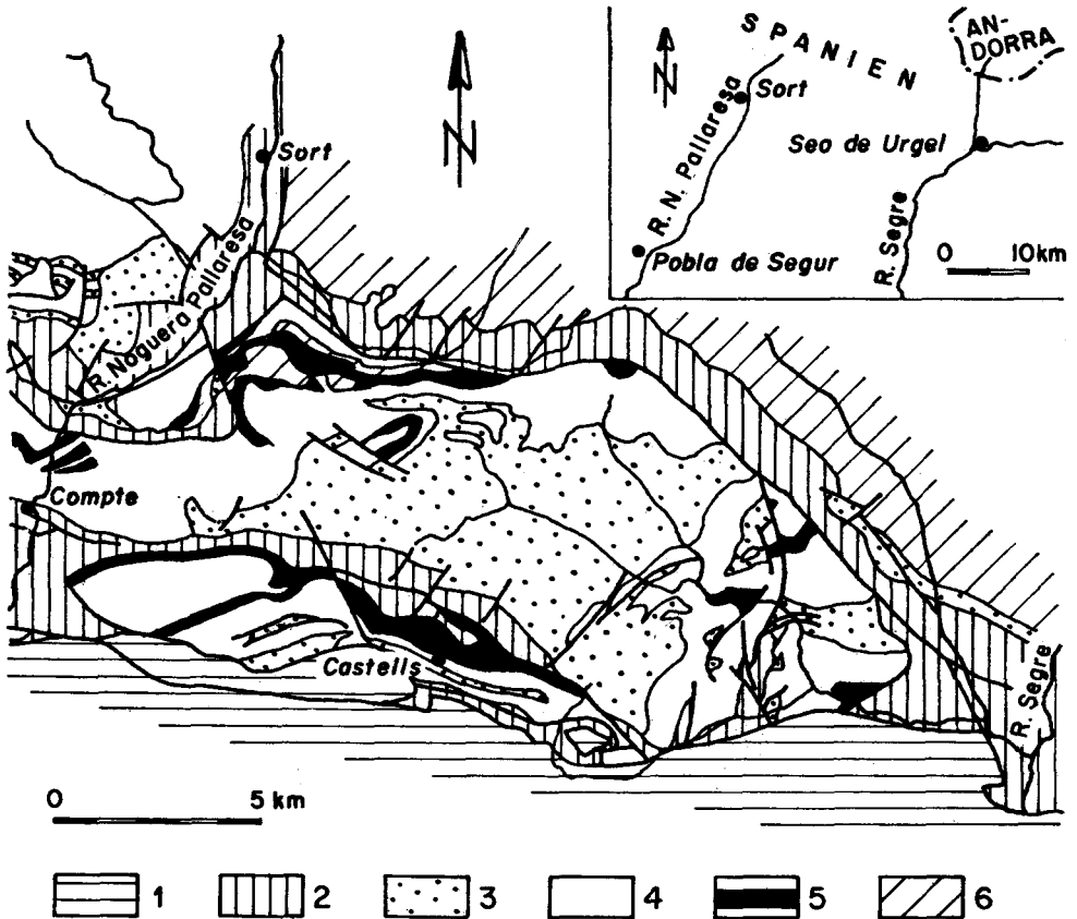
Abb. 1: Lageskizze und Geologie des Raumes zwischen Rio Segre und Rio Noguera Pallaresa (Geologie nach ZWART 1972) (1: Jura und Jüngerer, 2: Permo-Trias, 3: Karbon (überwiegend älter als Stephan), 4: Devon, 5: Silur, 6: Kambro-Ordovic)
