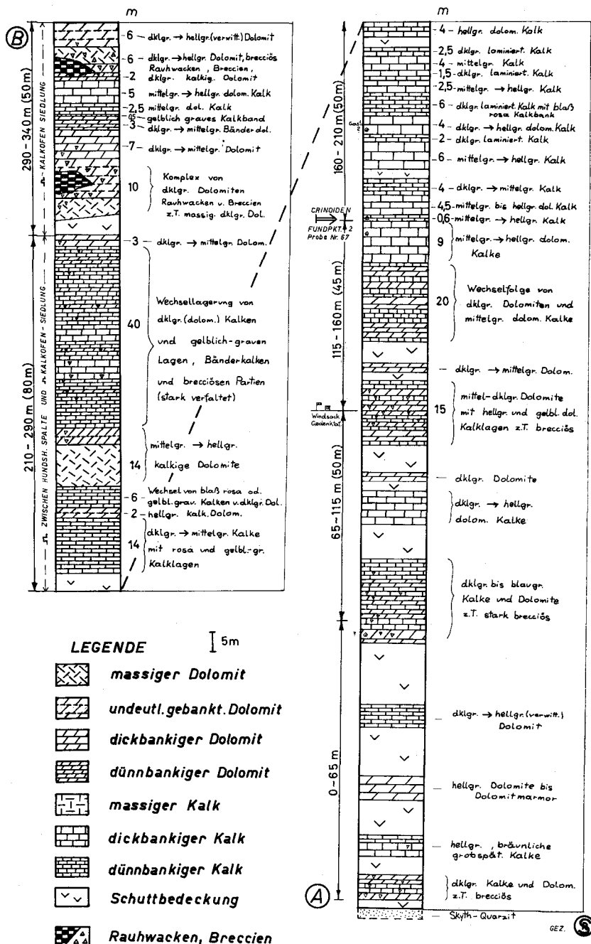
Taf. 3: Profil durch die Serien des Hexenberges nach einem Profilschnitt von Punkt A (200 m westlich des Sattels zwischen Hundsheim und Hainburg) und Punkt B (100 m SE der Kalkofen-Siedlung). Lage des Profilschnittes vgl. Taf. 1.
