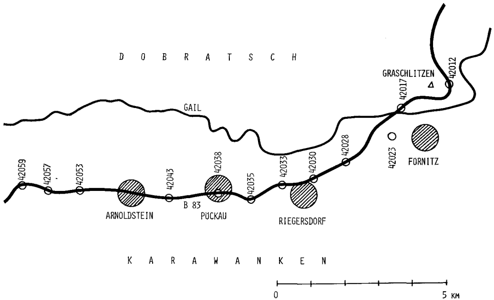
Abb. 1: Nivellementlinie Nr. 816 Villach — Thörl Maglern. Die bei den Nivellements 1952, 1964 und 1976 und in dieser Untersuchung verwendeten Höhenfixpunkte sind eingetragen.
