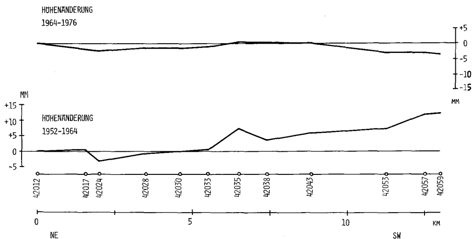
Abb. 2: Höhenvergleich der Nivellements 1952, 1964 und 1976. Ausgehend vom Höhenfixpunkt 42012 sind die Höhenänderungen für die Periode 1952–1964 und die Periode 1964–1972 in mm dargestellt.
