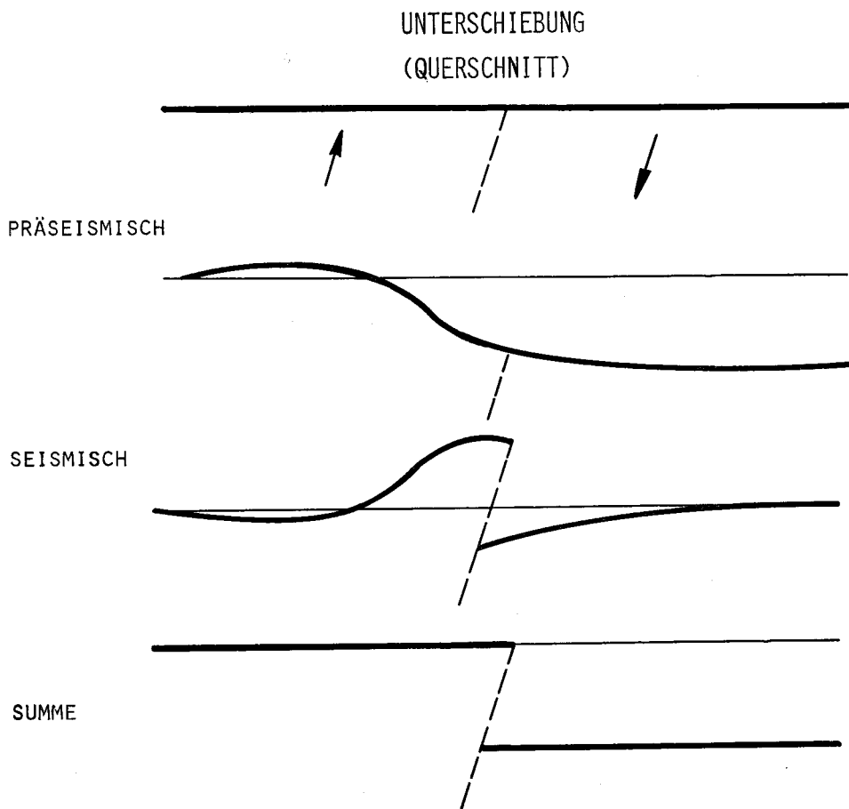
Abb. 3: Schema des elastischen „rebound“-Verhaltens an einer Unterschiebung [nach FITCH und SCHOLZ, 1971]. Die Pfeile geben die Richtung der langzeitlichen Bewegungen beiderseits der Verwerfung an. Die Oberfläche wird durch eine dicke Linie dargestellt. Die ursprünglich ebene Oberfläche (ganz oben) erleidet dadurch eine prä-seismische Deformation. Die durch ein Erdbeben ermöglichte seismische Gegenbewegung führt zur endgültigen Umgestaltung des Querschnitts (ganz unten).
