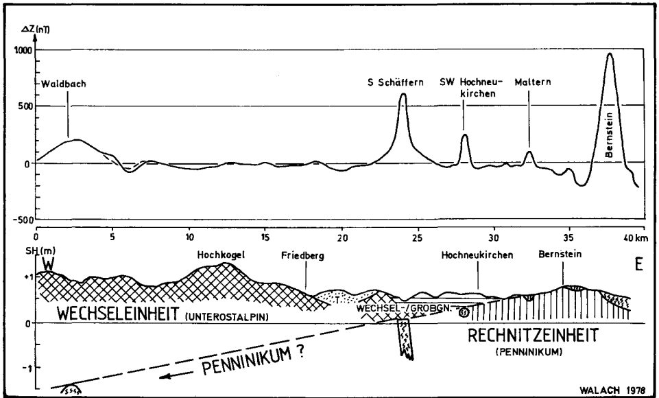
Abb. 7: Isanomalienprofil der magnetischen Vertikalintensität Waldbach — Bernstein aus G. WALACH (1977). Nimmt man an, daß die Anomalien durch Serpentine vom Typ Bernstein verursacht werden, so ergibt sich ein Abtauchen des Rechnitzer Penninikums mit 3—4° unter die unterostalpine Wechseleinheit, das bis in den Raum Waldbach verfolgbar ist.
