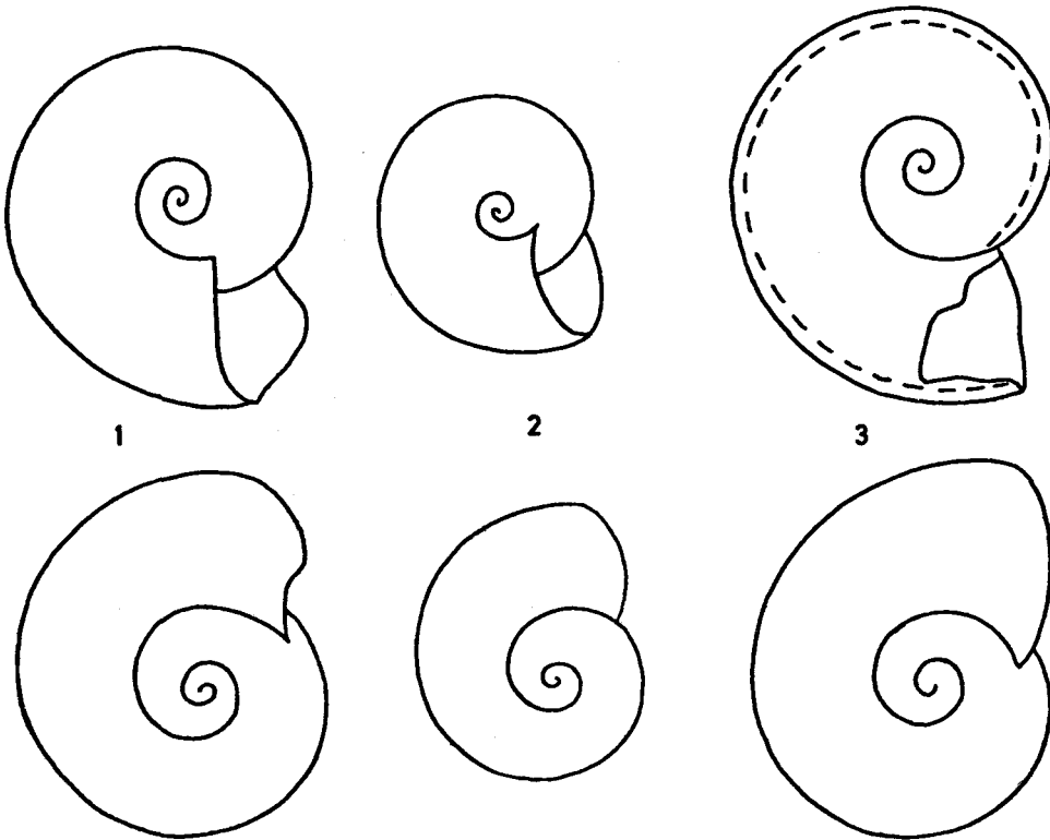
Abb. 4. Fig. 1. Gyraulus (Gyraulus) fuchsi (LORENTHEY), 13 : 1. P1d1. Fig. 2. Gyraulus (Gyraulus) micromphalus (FUCHS), 25 : 1. e (Unioschichten). Fig. 3. Gyraulus (Gyraulus) radmanesti (FUCHS), 13 : 1. c1.
