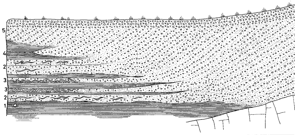
Abb. 5: Schematische Darstellung der Sedimente und Strukturen in einem Eisrandtasee mit hoher Sedimentationsrate.
