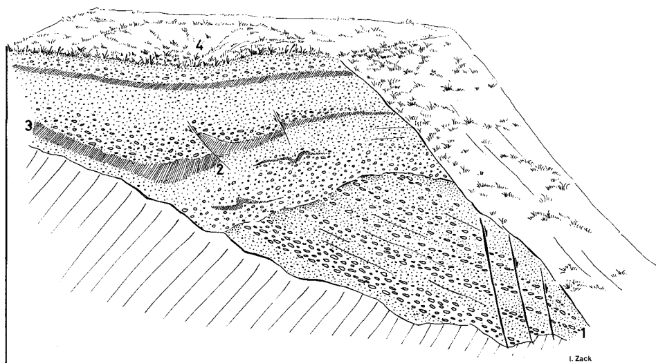
Abb. 6: Internstrukturen einer Eisrandterrasse (Wolfgangsee).
