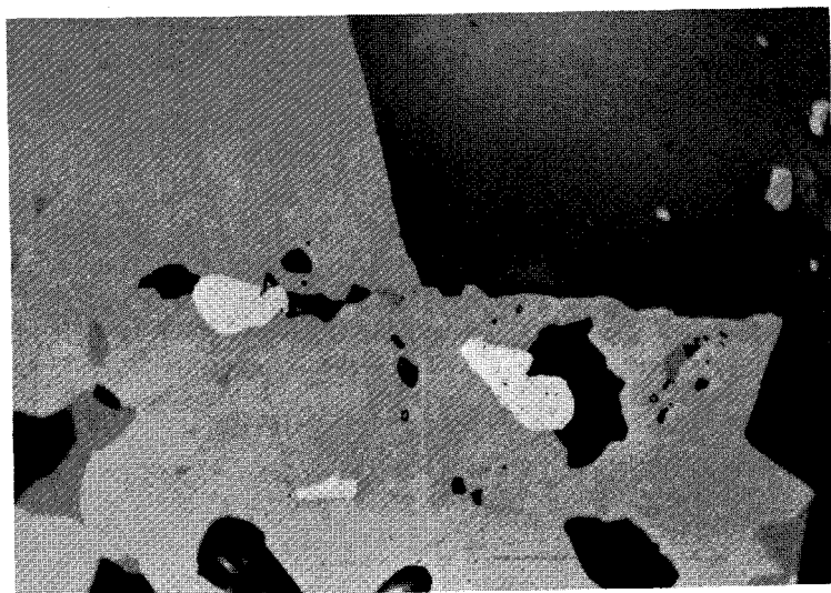
Abb. 32: Rammelsberg bei Goslar/Harz (Niedersachsen). 1. Teilsohle unter 10. Sohle, Pfeiler 271. Detail aus syngenetischem Bänderz mit vorherrschend Kupferkies (mittelgrau) und Gangart (dunkelgrau, fast schwarz, z. T. durch Innenreflexe aufgehell). Kupferkies enthält Einschlüsse von Gangart, etwas Bleiglanz (dunkelgrau) und gediegen Gold (hellgrau, fast weiß). Anschliff, Ölimmersion, Vergr.: 1000×
