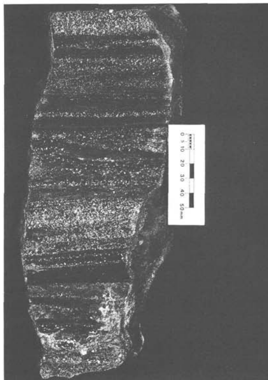
Abb. 12: Silberloch bei Ratten (Steiermark). Metamorph überprägte Wechselfolge von konkordanten Erz- und Nebengesteinslagen mit Schrägschichtung. Die Erzlagen sind vor allem durch idio-blastischen Pyrit (lichtgrau) und Magnetkies (ebenfalls lichtgrau) gegenüber den Nebenge-steinslagen (dunkelgrau – schwarz; darin jedoch auch Zinkblende, Bleiglanz etc.!) kenntlich.
