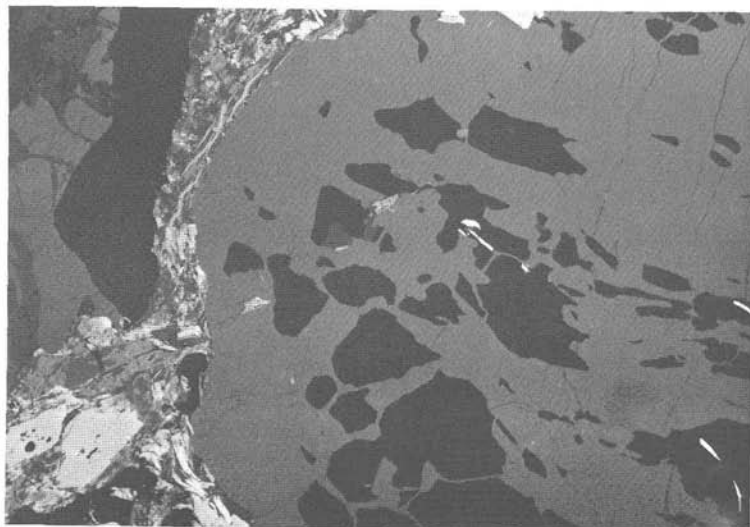
Abb. 24: Fuchs in Gstanach, Voral (Steiermark). Granat-Porphyroblast (mittelgrau) mit reichlich Einschluszügen („si“) bzw. Verdrängungsresten von Quarz (dunkelgrau), wenig Siderit (licht dunkelgrau) und kleinsten Graphit-Täfelchen (lichtgrau, fast weiß bis licht dunkelgrau ~ Reflexionspleochroismus!) weist randlich reichlich Graphit (linke Bildhälfte!), darin auch idio-blastischer Ilmenit (hellgrau; linke, untere Bildecke), auf. Anschliff, Vergr.: 75×
