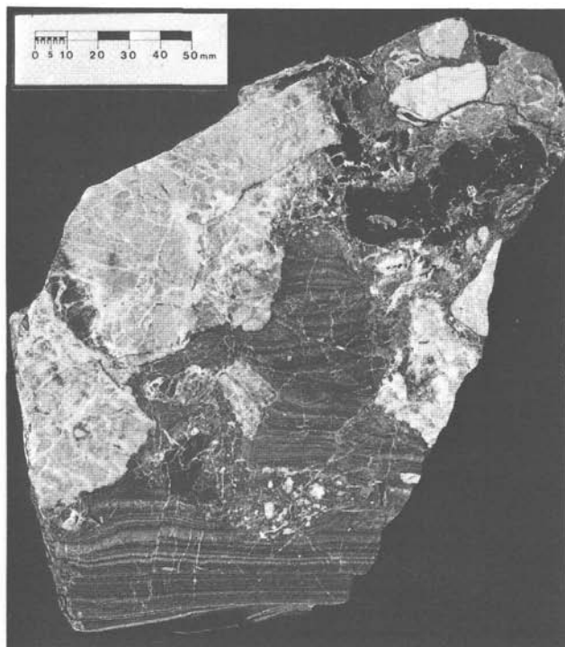
Abb. 6: Mežica, Graben-Revier, zentraler Teil, 12. Lauf. Ausschnitt aus Abb. 5. Detail mit Breccie im feinschichtigen Erz-Sediment (Zinkblende-Bleiglanz-Dolomit-Rhythmit), das Load-casts aufweist. Im Hangenden findet sich eine größere Partie von sammelkristallisiertem Bleiglanz.
