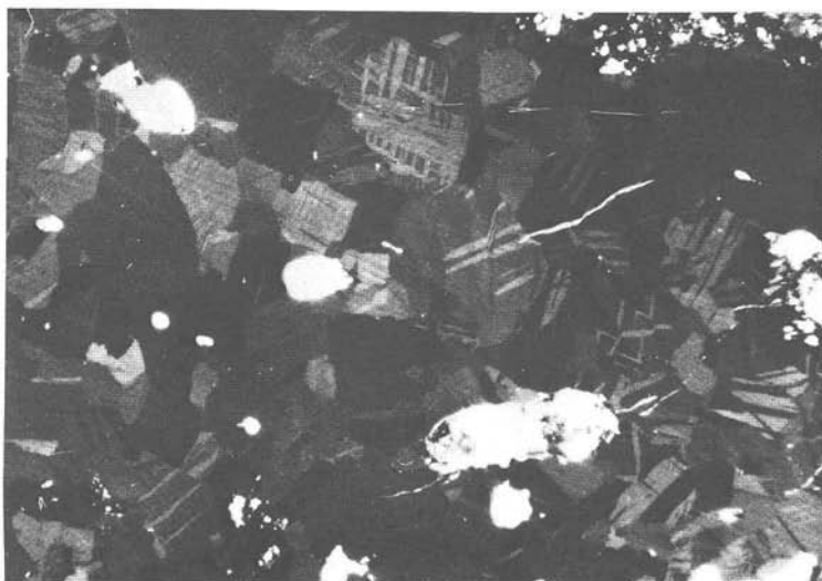
Abb. 22: Panzendorf (Osttirol). Ausschnitt aus körnigem Rekristallinat von vorherrschend Kupferkies, etwas Magnetkies (durch Anisotropie-Effekte stark aufgehell – weiß) und wenig Gangart (durch Innenreflexe stark aufgehell – weiß). Kupferkies hat sogar in den körnigen Rekristallinaten die typischen oleanderblatt- bis lanzettförmigen Umwandlungslamellen von Hochtemperatur-Kupferkies ausgebildet. Anschliff, Vergr.: 115 \times , Polarisatoren +
