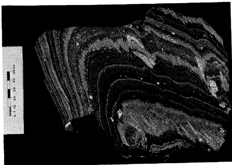
Abb. 31: Rammelsberg bei Goslar/Harz (Niedersachsen). 11. Firste, Kammer 284, + 1600. Syngenetisches „Bänderz“ mit deutlich ausgebildeter Biegesccherfalte.
