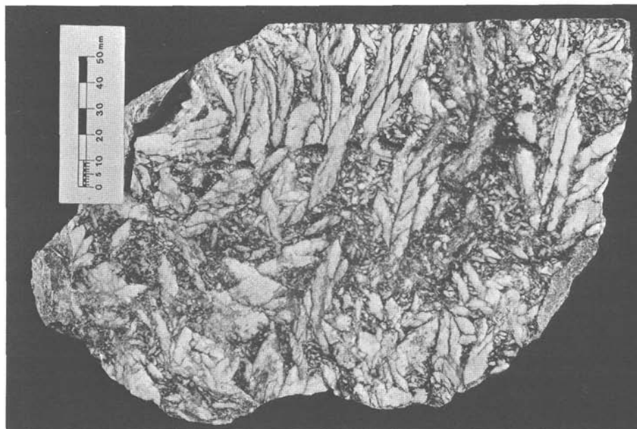
Abb. 4: Millstätter Alpe/Radenthein (Kärnten). „Pinolitmagnesit“. Grobkörniger, unreiner Magnesit-Marmor, bestehend aus aufgesproßten, an Pignolien erinnernde Magnesit-Porphyroblasten bzw. -Idioblasten in stark pigmentierter Matrix.
