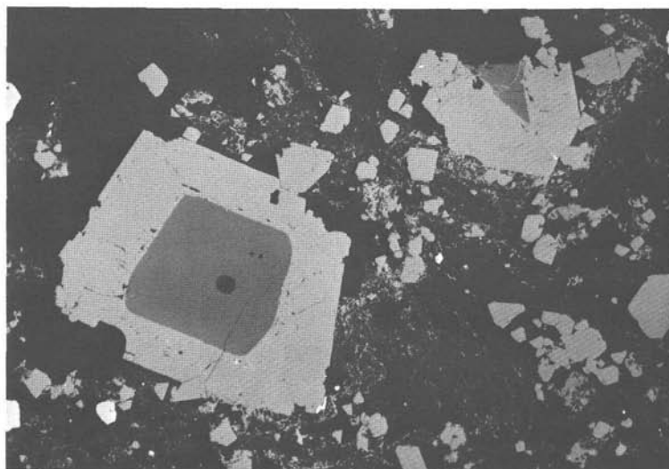
Abb. 28: Arzwaldgraben, Waldstein (Steiermark). Baryt-Gangart (fast schwarz), darin reichlich idiomorphischer Magnetit (mittelgrau), der im Zentrum Chromit (dunkelgrau) als Einschluß, z. T. in vergleichbarer Kristallform, aufweisen kann. Neben kleinen Magnetit-Idioblasten finden sich feinkörnige Rutil-Aggregate und -Züge (ebenfalls mittelgrau) sowie örtlich etwas Pyrit (lichtgrau) in der Baryt-Gangart. Anschliff, Vergr.: 150×
