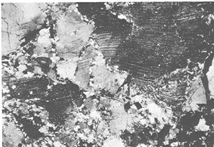
Abb. 33: Löffel-Graben, Voralu (Steiermark). Ausschnitt aus altem, sericitisiertem, postkristallin stark deformiertem und zerbrochenem Albit-Korn (undulöses Auslöschcn, verbogene und zerbrochene feinlamellare Albit-Zwillingslamellen!) mit Rekristallisation von Albit in den zerriebenen Partien. Stellenweise findet sich kleiner idiomorpher Arsenkies (schwarz). Dünnschliff, Vergr.: 10X, Polarisatoren +
