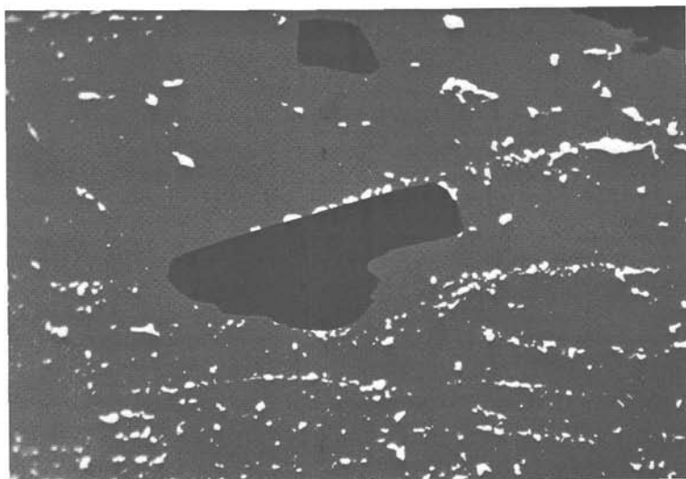
Abb. 34: Löffel-Graben, Voralu (Steiermark). Zinkblende (dunkelgrau), darin etwas Gangart (schwarz), weist Entmischung von Magnetkies (hellgrau) auf. Anschliff, Ölimmersion, Vergr.: 375X
