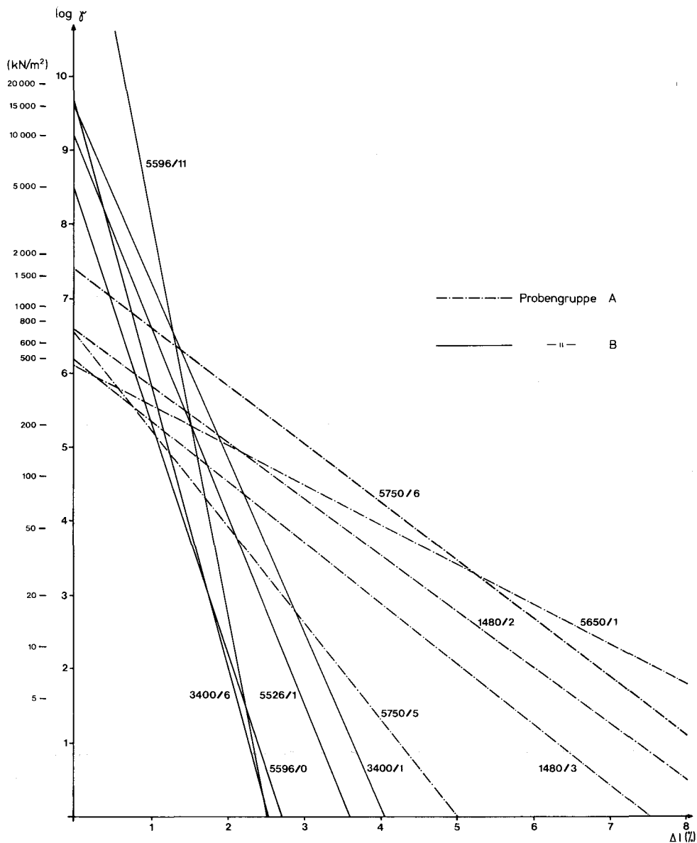
Abb. 5: Dehnungs/Spannungs-Diagramm. Abhängigkeit der Quelldehnung von der im Versuch aufgetragenen Normalspannung.
