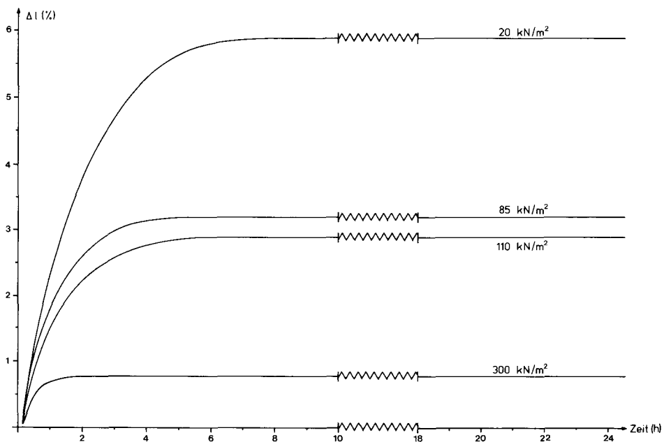
Abb. 3: Quelldehnung einer Probe aus den OSM-Mergeln bei km 5,65 bei verschiedener Belastung.
