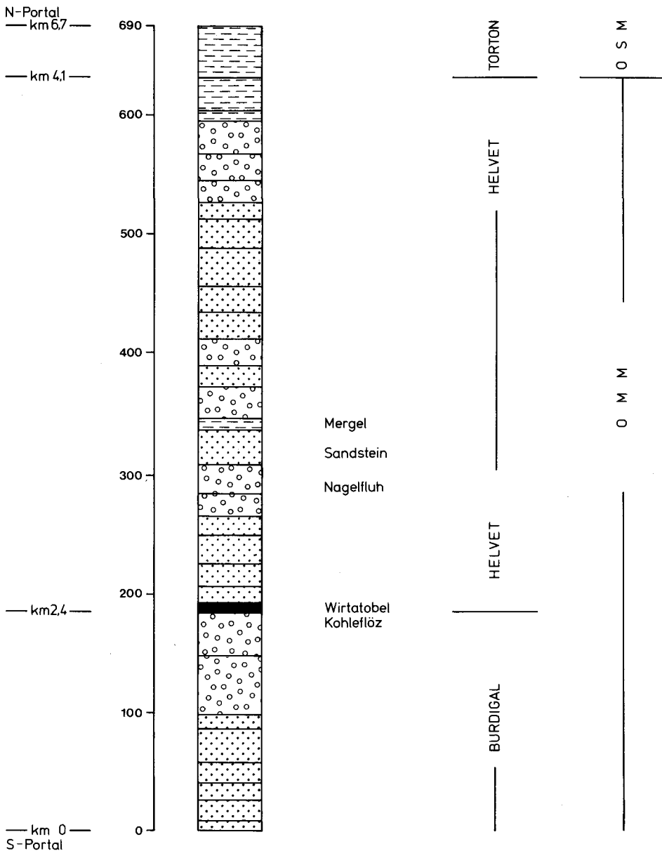
Abb. 1: Idealisiertes Säulenprofil der Serien der OMM und OSM (Eggenburg bis Baden) entlang der Pfändertunnel-Strecke.
