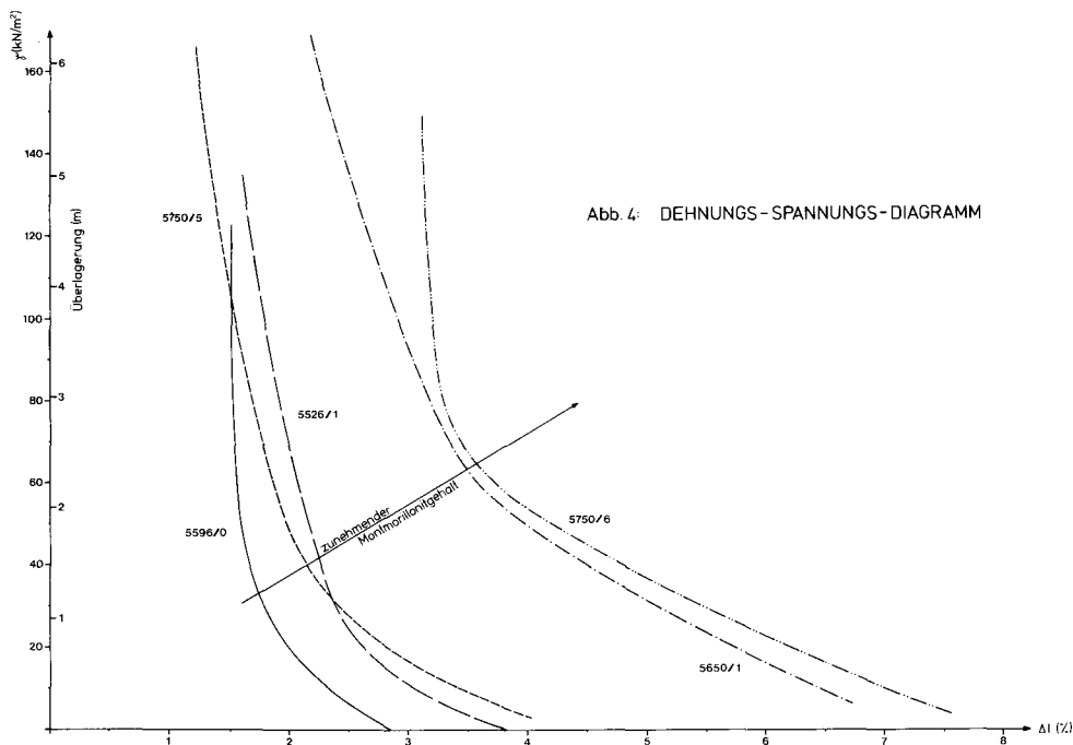
Abb. 4: Abhängigkeit der Quelldéhnung von Belastung und Montmorillonit-Gehalt.
