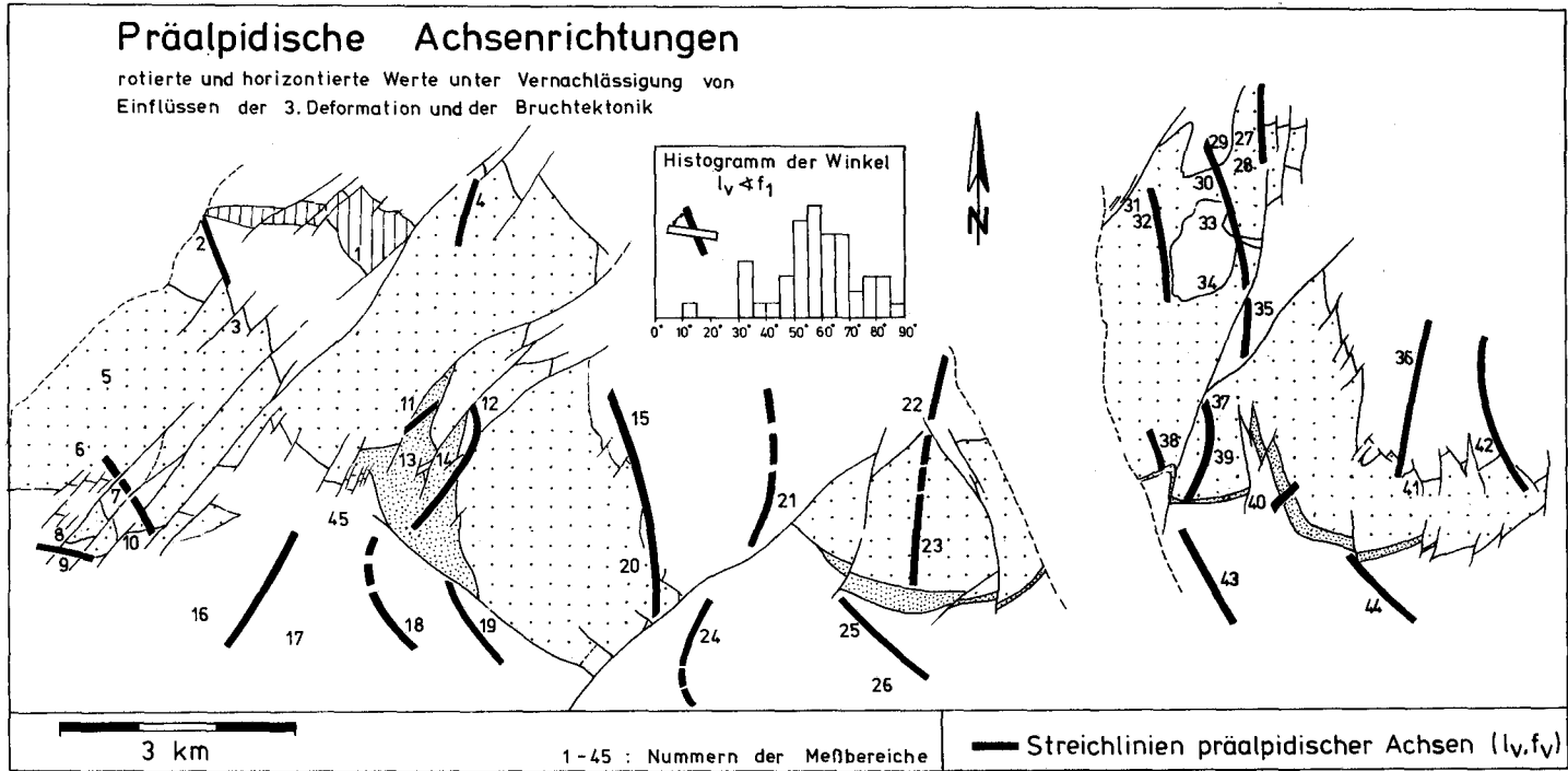
Abb. 5: Präalpide Achsenrichtungen ( l_v , f_v ) im Bereich der Kellerjochgneise und angrenzender Gebiete. weit gepunktet: Kellerjochgneiss eng gepunktet: Albit-Chlorit-Phyllonitserie schraffiert: oberostalpine Quarzporphyre
