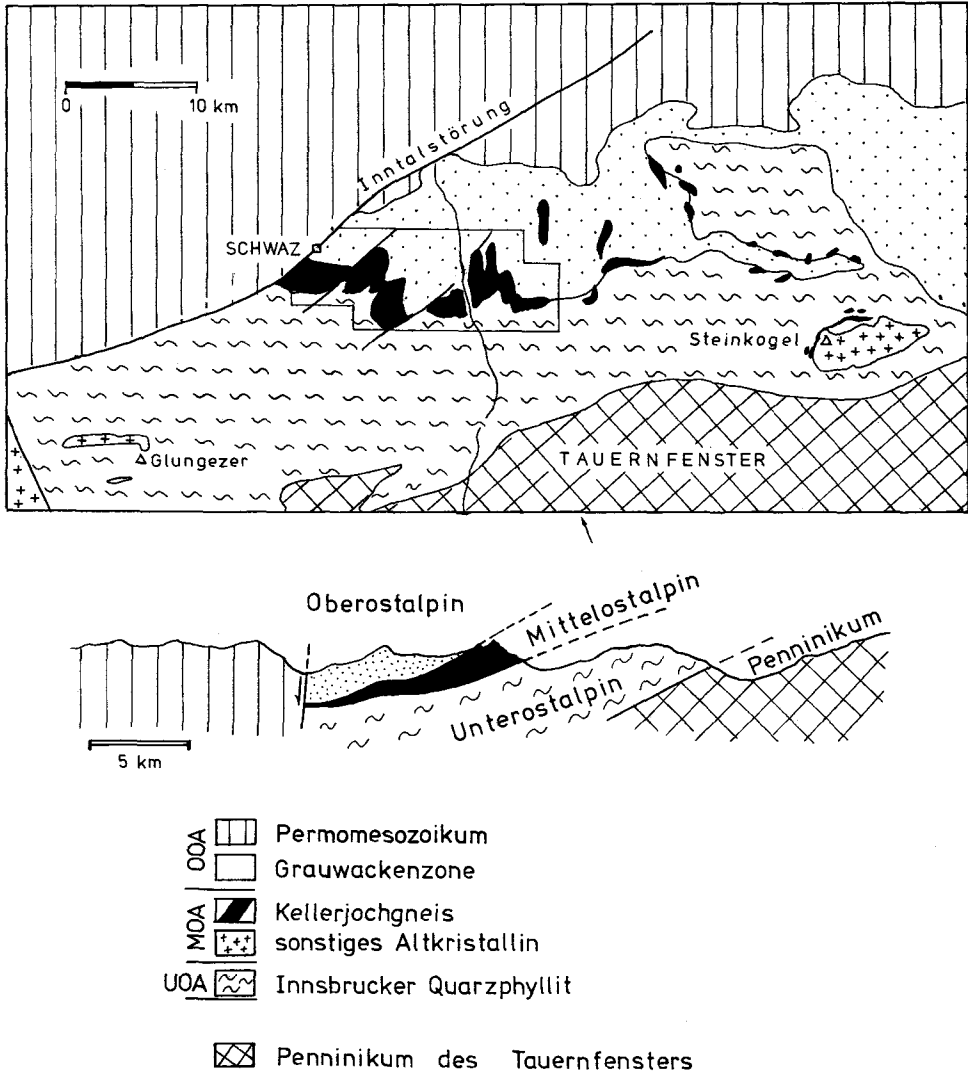
Abb. 1: Geologische Übersicht zur Position der Kellerjochgneis-Decke nördlich des Tauernfensters.
