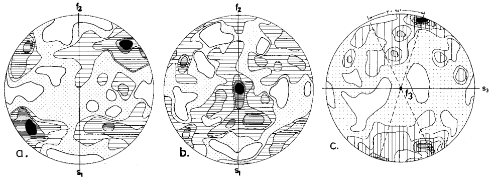
Abb. 13: Wichtigste Quarzregelungstypen im Untersuchungsgebiet.
