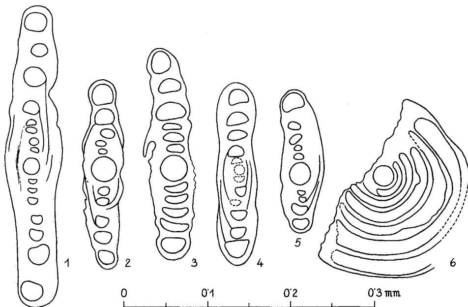
Abb. 10: Angulodiscus aus dunkelgrauem Kalk der Obertrias, Unterkarn, Zone des Trachyceras aon ; S 8. Linke Seite des Lissar-Flusses gegenüber dem Ralphu-Gletscher bei Byans, Zentral-Himalaya. Fig. 1, 4, 5: Angulodiscus tenuis KRISTAN Fig. 2, 3: Angulodiscus fragilis (LIEM) Fig. 6: Angulodiscus sp. – schräger Schnitt von einer der beiden vorhergehenden Arten.
