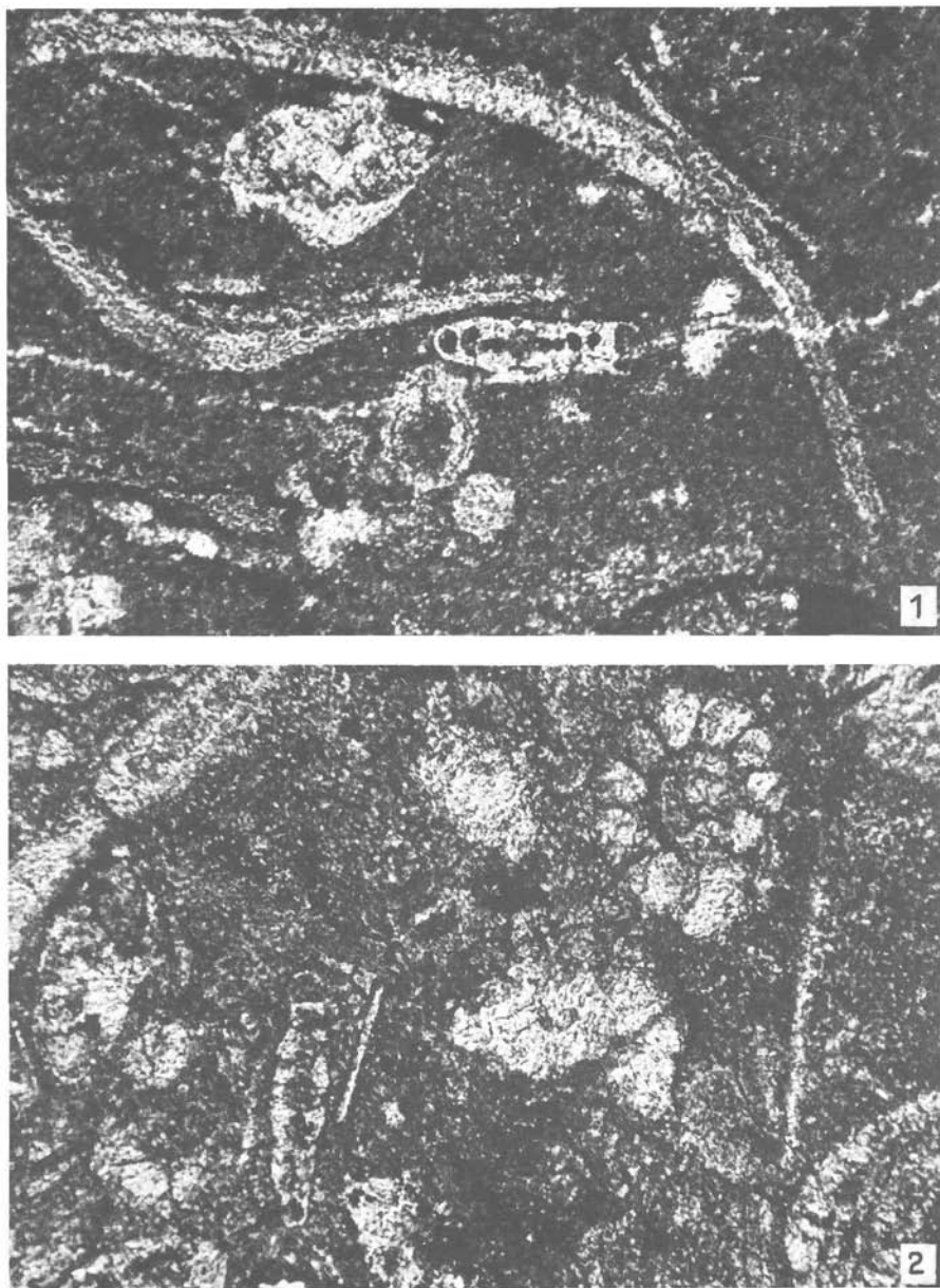
Abb. 3. Beispiel der Mikrofazies des unterkarnischen Kalkes vom Lissartal bei Byans. Die pseudomikritischen, Pellets enthaltenden Kalke führen vor allem Foraminiferen – hier in beiden Figuren Schnitte von Diplotremina und Angulodiscus fragilis (LIEM) –, sonst ferner häufig Echinodermenreste, Bivalvenschalen, selten auch Globochaete alpina LOMBARD.
