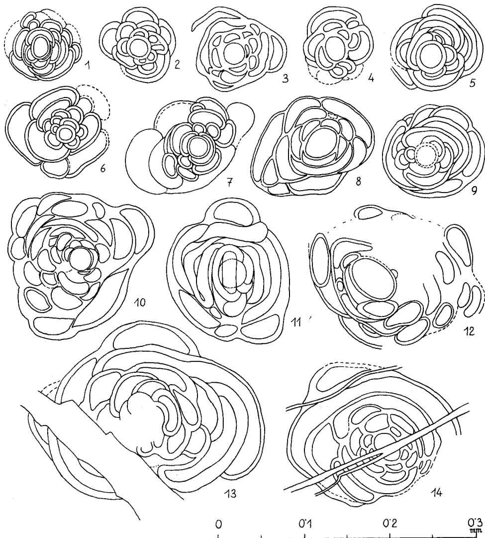
Abb. 5: Meandrospira dieneri n. sp.
