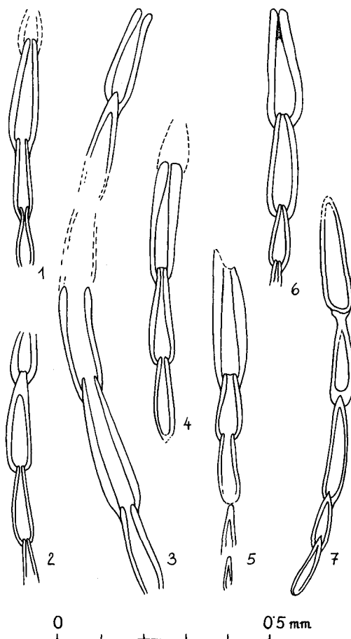
Abb. 8: Nodophthalmidium vujsici (UROŠEVIĆ & GAZDZICKI) Mitteltrias, Ladin, Lumachelle mit Daonella indica . Dogkwa Aur, Hop Gadh, Hundes, Zentral-Himalaya. Fig. 1, 2, 4–6: S 24C; Fig. 3: S 24B; Fig. 7: S 24A. Verschiedene Schliff-Schnittlagen, Anfangsteil nirgends getroffen.
