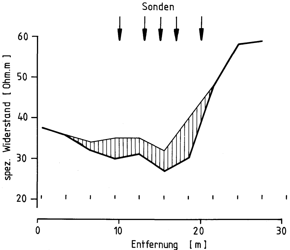
Abb. 6: Auswirkungen der Bentonitinfiltration auf den gemessenen Formationswiderstand (dünne Linie Meßwerte vor, dicke Linie nach der Infiltration); Dipol-Dipol-Kartierung, Elektrodenabstand a = 3 m, Dipolseparation n = 5 .
