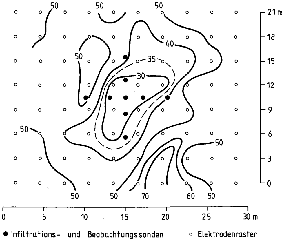
Abb. 7: Isoohmenplan des Testfeldes nach Abb. 5 nach erfolgter Infiltration (Dipol-Dipol-Kartierung, a = 3 m, n = 5 ).
