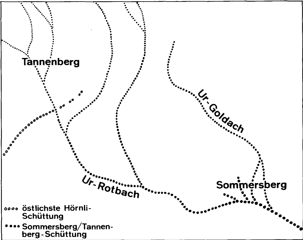
Abb. 9: Die mittelmiozäne Sommersberg-Tannenberg-Schüttung.
