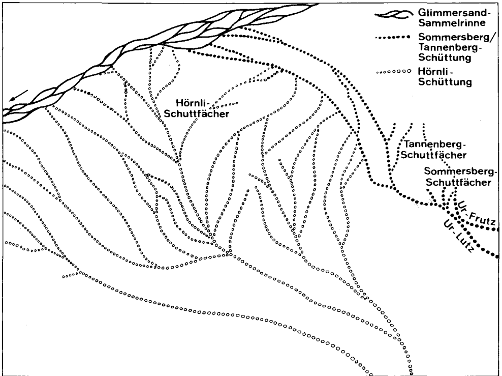
Abb. 8: Die mittelmiozänen Schüttungen in der NE-Schweiz.
