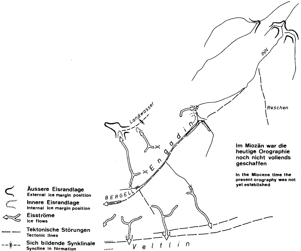
Abb. 6: Eisabfluß aus dem Bergell-Bernina-Gebiet gegen N, NE, und S.
