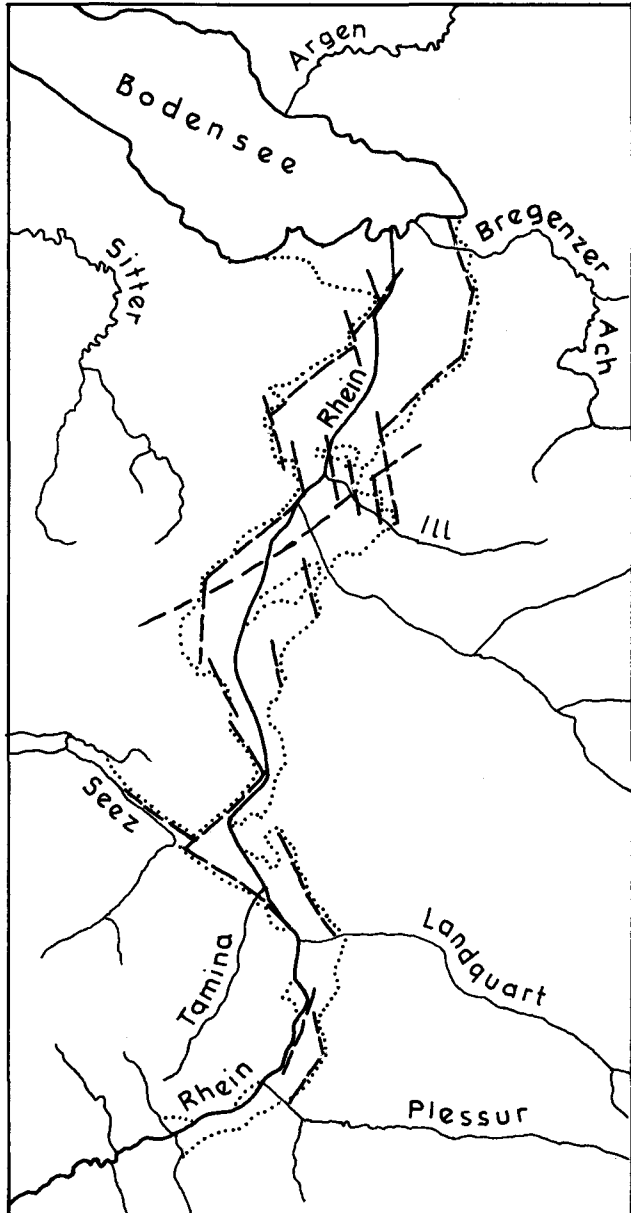
Abb. 16: Die strukturell verschiedenen Abschnitte des Alpen-Rheintals.
