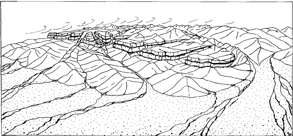
Abb. 10: Die westlichen Ostalpen, aufgeschoben auf penninischen Flysch zur Zeit der Schüttung von Gaiskopf-Fallenbach- und Gäbris-Schüttung im jüngeren Oligozän-älteren Miozän.
