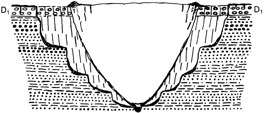
Abb. 2: Aufgrund neuer geologischer und palynologischer Daten umgedeutetes schematisches Querprofil durch ein altes Gletschertal in der Molasse, das zur Bildung des Höheren Deckenschotters D 1 führte.
