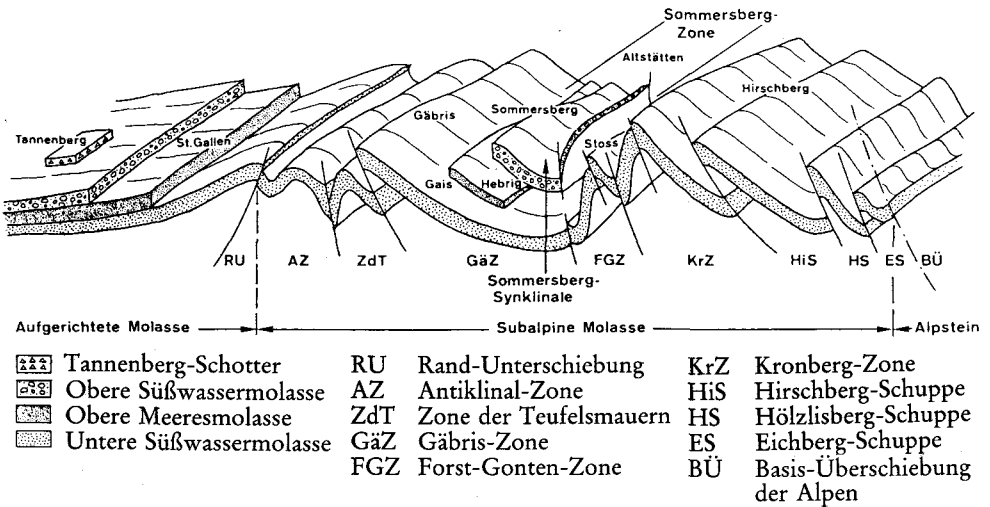
Abb. 15: Struktur-Schema der gestauchten st. gallisch-appenzellischen subalpinen Molasse, nach H. HEIERLI 1984 und S. BERLI 1985, leicht modifiziert.
