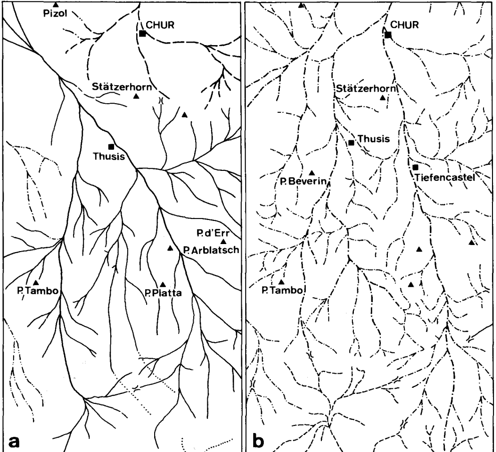
Abb. 4a, b: Darstellung der Quelläste im zentralen Einzugsgebiet des heutigen Alpen-Rheintales im Oligozän (a) und im mittleren Miozän (b); nach R. STAUB 1952.
