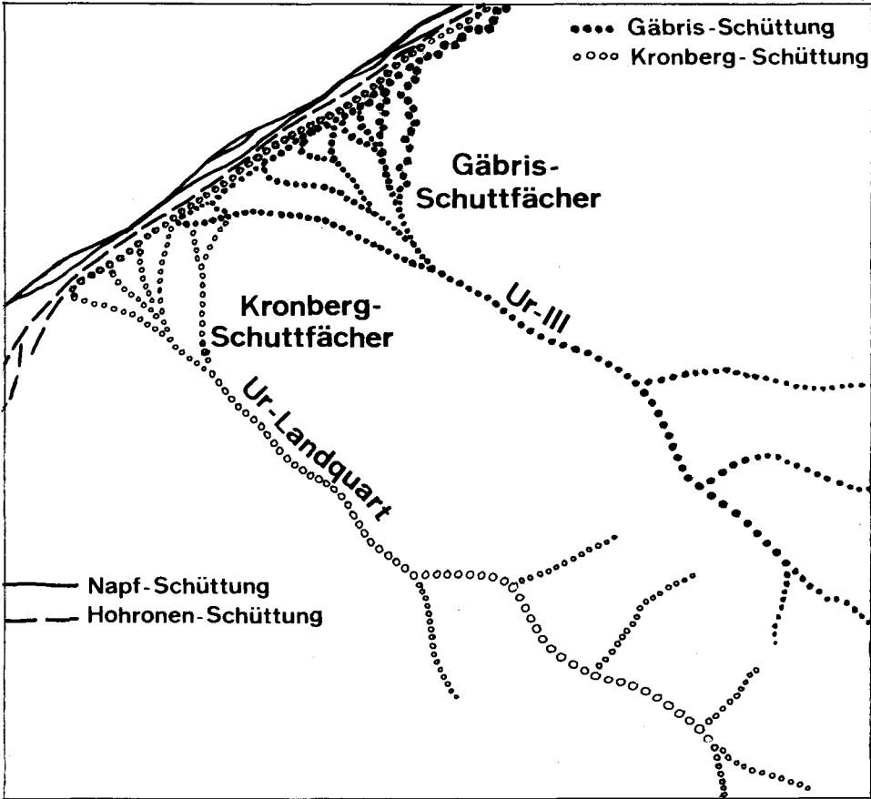
Abb. 3: Die jungoligozänen bis frühmiozänen Schüttungen in der NE-Schweiz.
