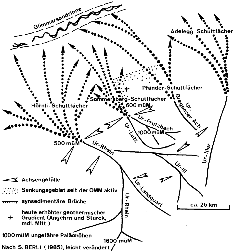
Abb. 7: Die Flußsysteme der Nordostschweiz im mittleren Miozän, vor 15–10 Millionen Jahren.
