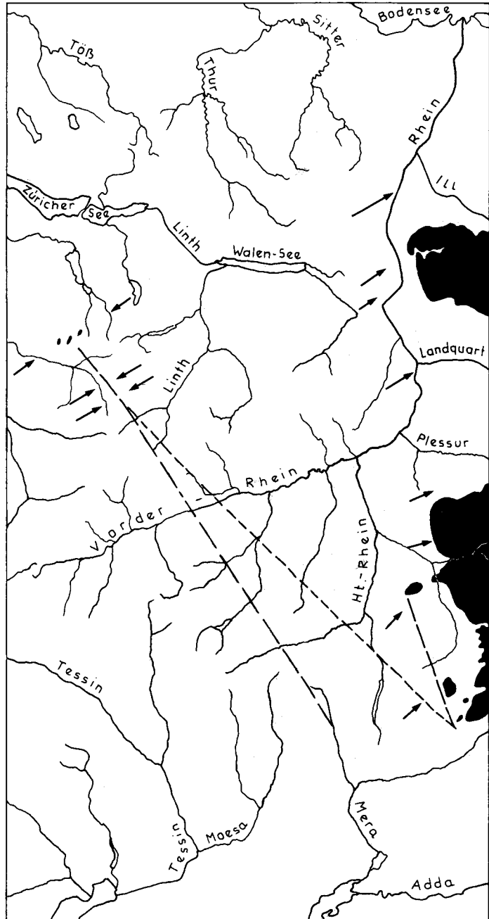
Abb. 14: Der Westrand der Ostalpinen Decken (schwarz) und die gegen NW-orientierte Bahn der Iberger Klippen in der östlichen Zentralschweiz (kurze Strichel) durch die helvetische Depression (gegenseitige Pfeile). Durch das seitliche Abgleiten (Pfeile) wurde der Westrand der Ostalpinen Decken (lange Strichel) gegen Osten verschoben.
