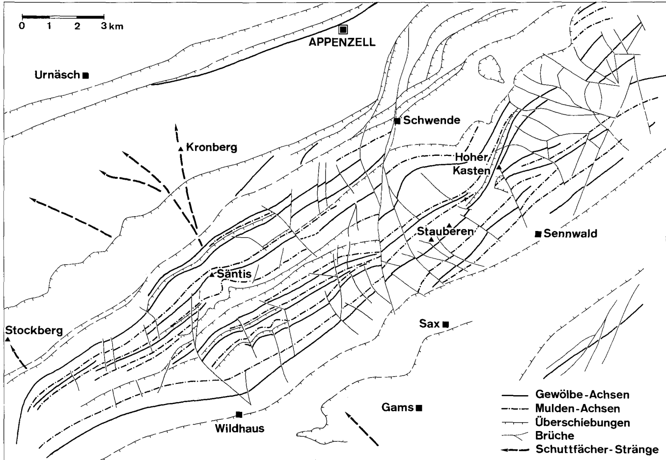
Abb. 13: Geologische Strukturen im Säntis-Gebirge nach Th. KEMPF 1966 und H. EUGSTER et al. 1982, ergänzt.
