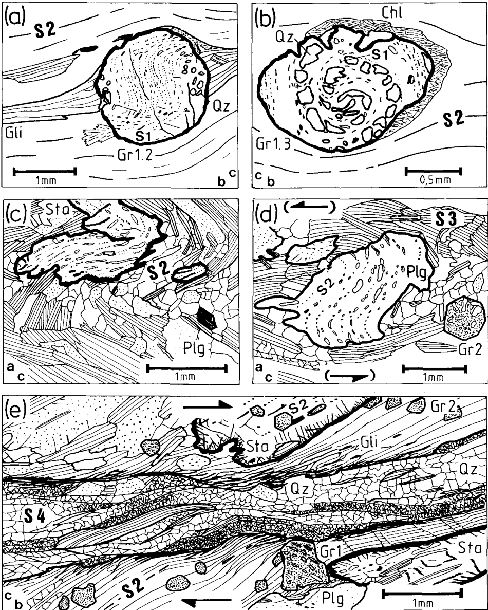
Abb. 2: (a) Synkristallin rotierter Granat Gr1.2 mit beginnender Druckschattenbildung. Rotation des Blasten um etwa 90^\circ um Rotationsachse parallel a; Rotations-, Bewegungs- und Scherrichtung liegen parallel b. (b) Synkristallin rotierter Granat Gr1.3 mit Druckschattenspirale. Rotation des Blasten um ca. 360^\circ um Rotationsachse parallel a; Rotations-, Bewegungs- und Scherrichtung liegen parallel b. (c) Staurolith überwächst D3-Crenulation. (d) Plagioklas überwächst D3-Crenulation; an den Faltenflanken beginnende Crenulationsschieferung S3 mit leichter Scherung parallel c. (e) S4-Scherbahn durchschlägt und versetzt S2-Gefüge. Abkürzungen siehe Abb. 3.
