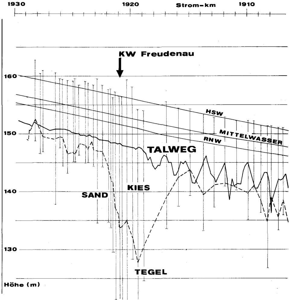
Abb. 2: Schematischer geologischer Längenschnitt längs der Donau im Bereich der Schwechatzer Mulde, 500fach überhöht: strichliert — Kiesbasis am rechten Ufer, im Liegenden Sande und schließlich „Tegel“.
