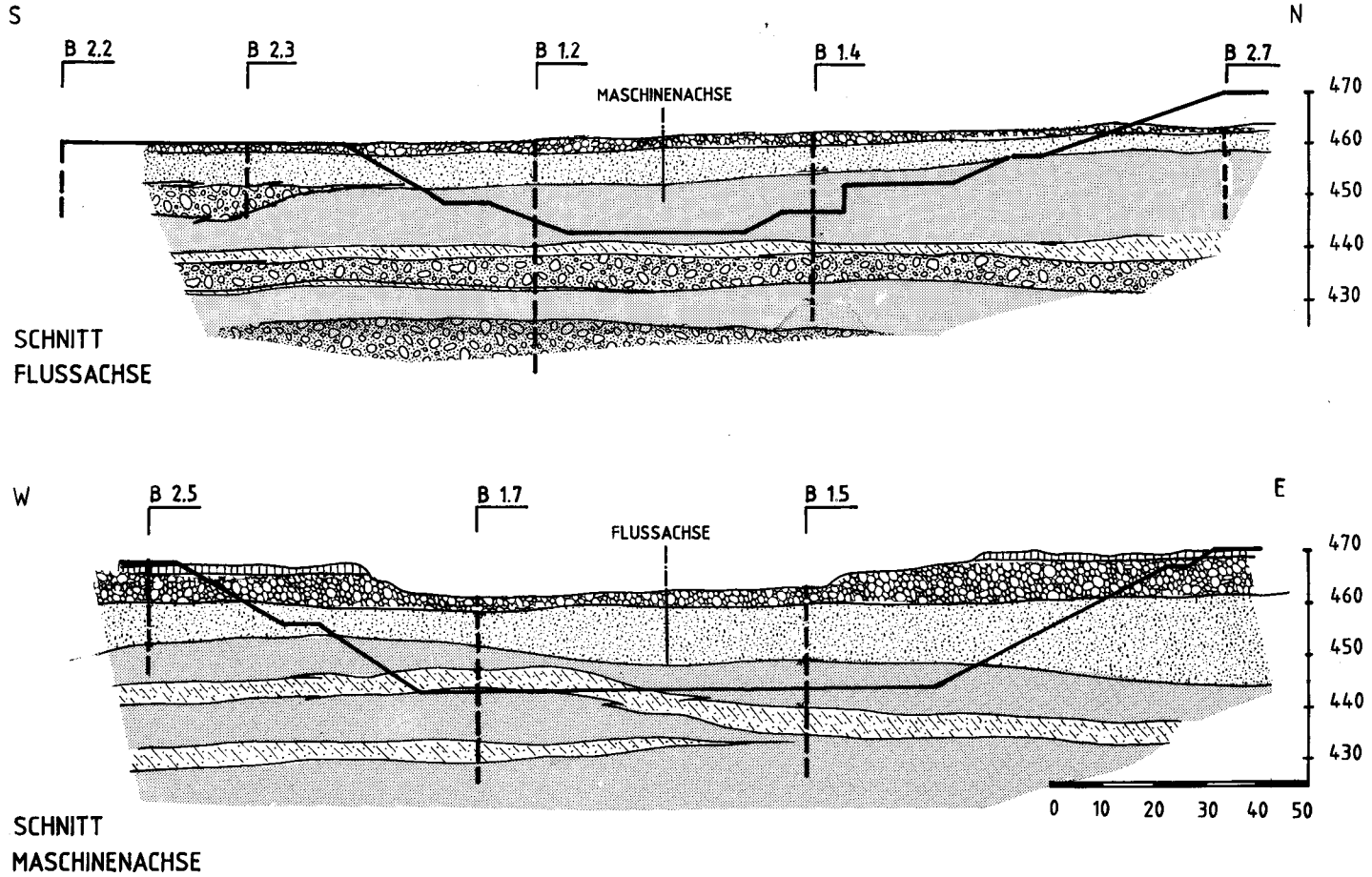
Abb. 2: Vereinfachter geologischer Schnitt entlang der Fluß- und der Maschinenachse [Legende siehe Abb. 7].
