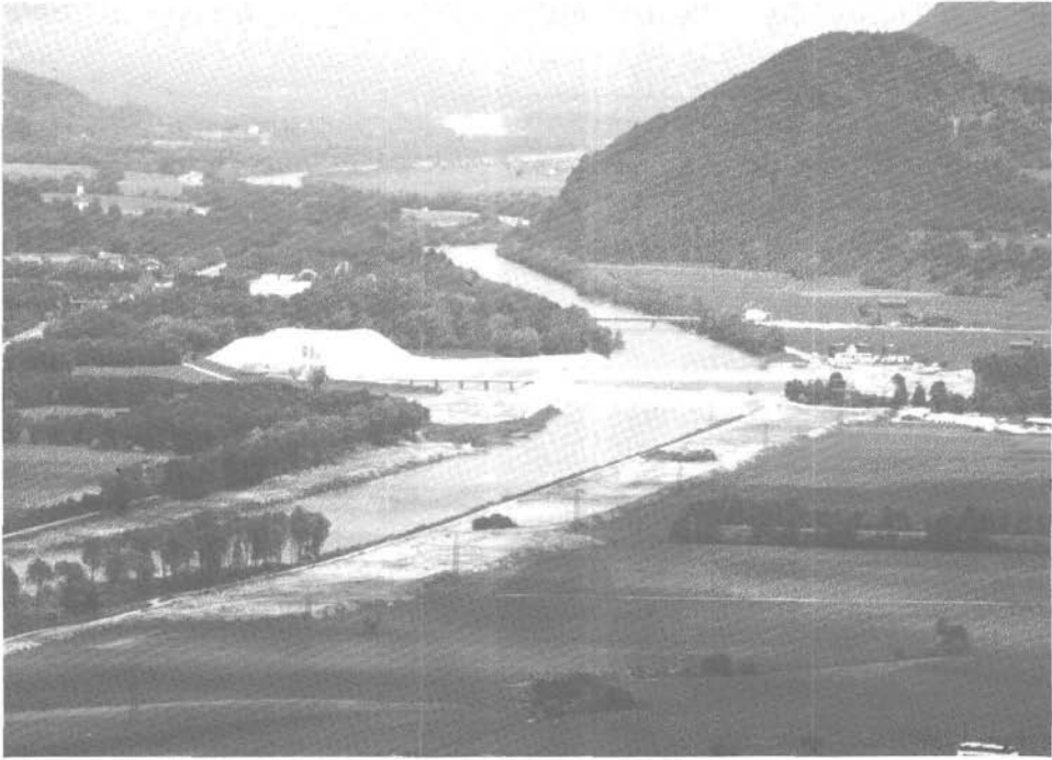
Abb. 3: Übersicht über den Baustellenbereich, Blickrichtung Norden.
