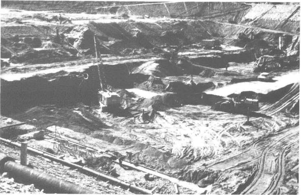
Abb. 13: Übersicht über die Baugrube bei Erreichen der tiefsten Aushubsohle.
