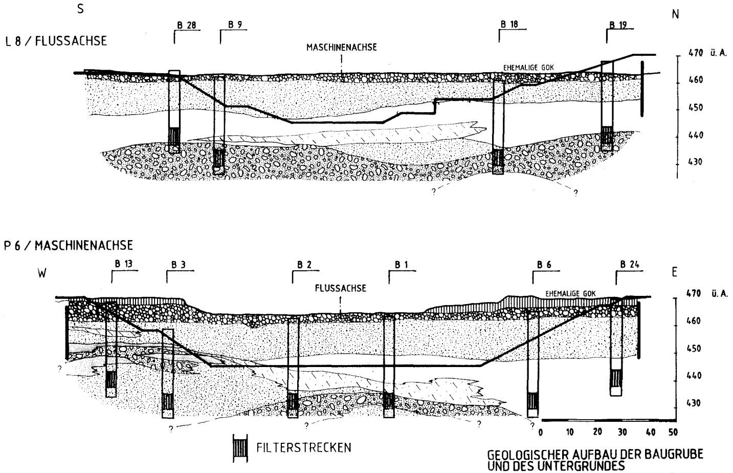
Abb. 6: Schematischer Längs- und Querschnitt in Baugrubenmitte mit Verteilung der Brunnen.
