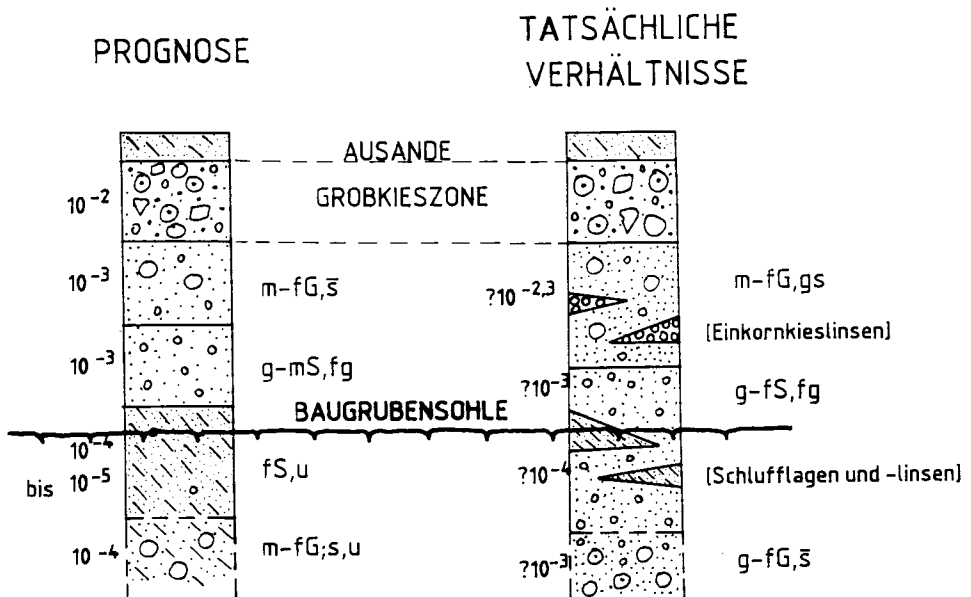
Abb. 15: Schematischer Vergleich Prognose — tatsächliche Verhältnisse.
