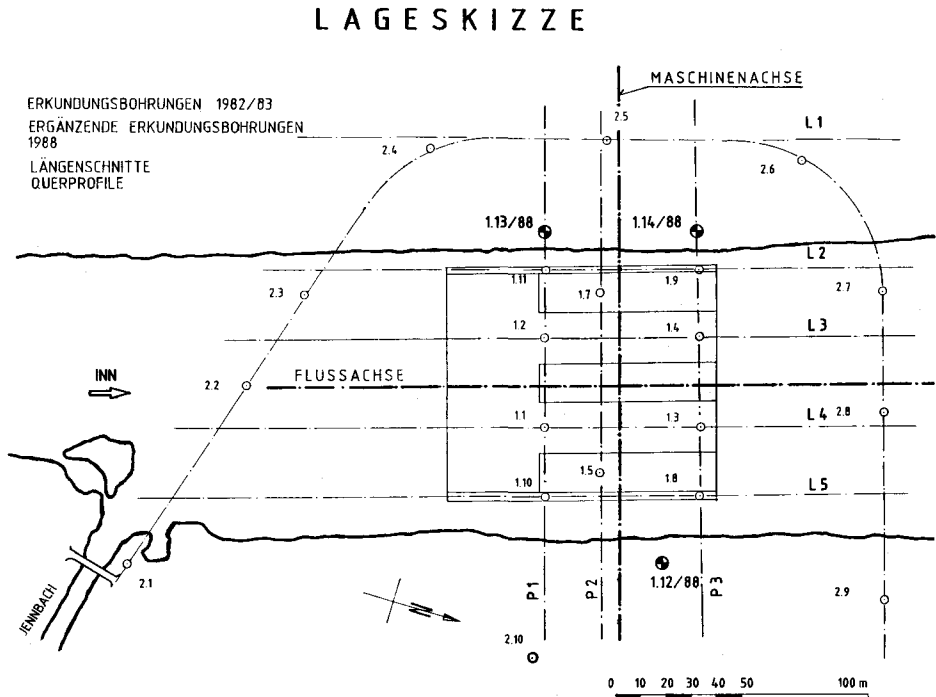
Abb. 1: Lageskizze des Hauptbauwerkes [ca. 1.5 km NW von Ebbs] und Anordnung der ausgeführten Erkundungsbohrungen [B 1.1 — 1.11 — Hauptbauwerk; B 2.1 — 2.10 — Baugrubenumschließung].
