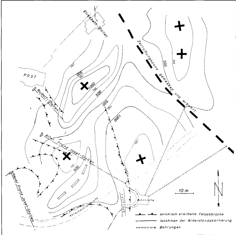
Abb. 2: Ergebnisse der geoelektrischen und refraktionsseismischen Messungen: ermittelte Isoohmen der Widerstandskartierung und die Richtung zweier Bohrungen, die die Zerrüttungszone erreichten. Ferner die seismisch ermittelten Kanten von Felsabbrüchen unter den Lockermassen des Hanges.
