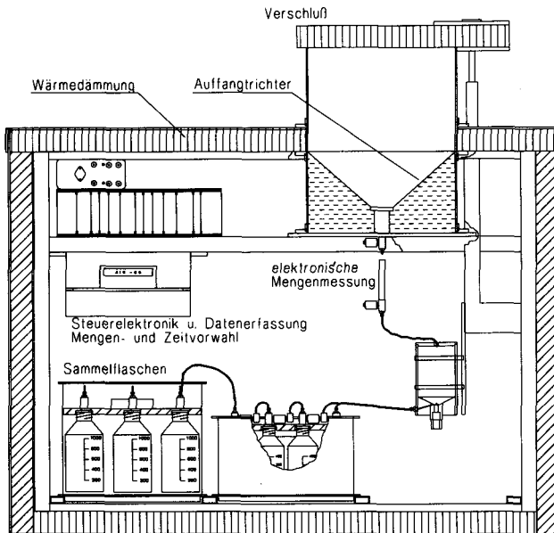
Abb. 11: Niederschlagsprobensammler zur Untersuchung von Einzelereignissen (Prototyp an der BVFA Arsenal). Der Sammler erlaubt die fraktionierte Sammlung von Proben wäh- rend eines Niederschlagsereignisses mit Vorwahl der Sammelzeit bzw. der Sammel- menge. Das Gerät schaltet sich mit Beginn bzw. Ende des Niederschlagsereignisses auto- matisch ein bzw. aus.
