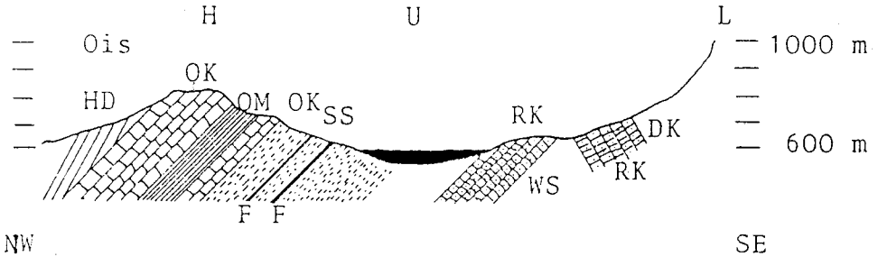
Abb. 2: Geologisches Profil vom Ois-(Ybbs)-tal über die Hinterleiten (H), den Untersee (U) zum Lärchenstein (L). Höhe und Länge 1:75. WS: Werfener Schichten OK: Opponitzerkalk RK: Gutensteinerkalk OM: Opponitzer Mergel SS: Sandstein und Schiefertone HD: Hauptdolomit F: Flöze DK: Dachsteinkalk Nach GÖTZINGER 1910
