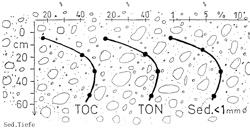
Abb. 7: Vertikalverteilung von POM in den Bettsedimenten: x-Achse: relativer Anteil von TOC, TON und Korngrößenklasse < 1 \text{ mm } \varnothing y-Achse: Sedimenttiefe (cm)
