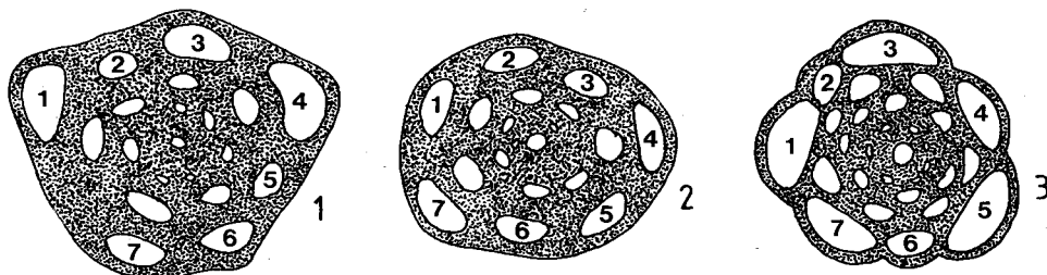
Abb. 7: Kammeranordnung bei verschiedenen Arten der Gattung Septuloculina EL-NAKHAL. 1. S. angulata 2. S. rotunda 3. S. cretacea n. sp.
