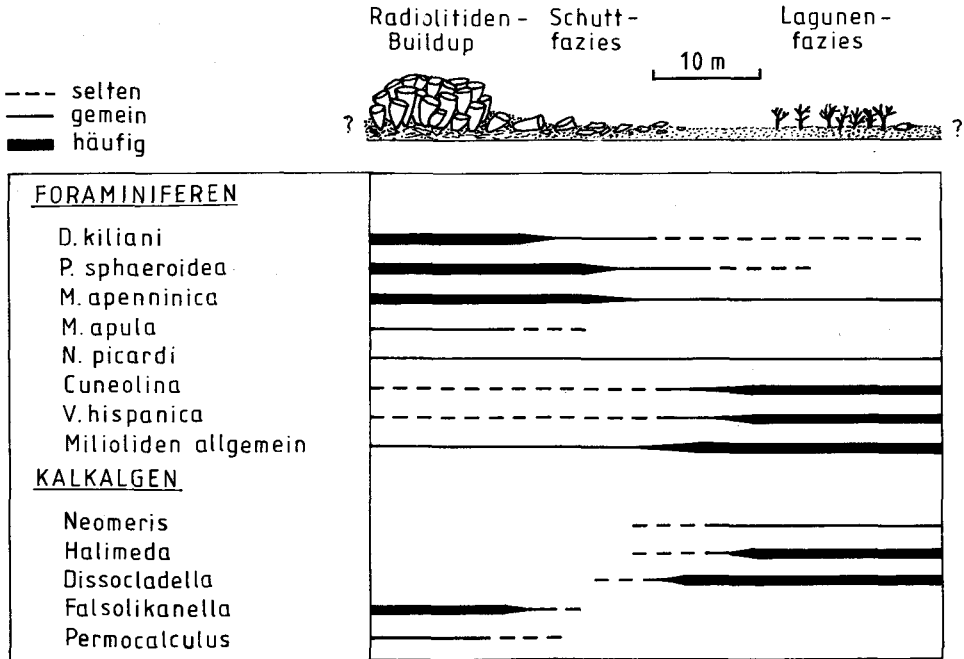
Abb. 10: Qualitative und quantitative Verbreitung der Benthosforaminiferen und Kalkalgen in der Pleitzachalm-Gosau.
