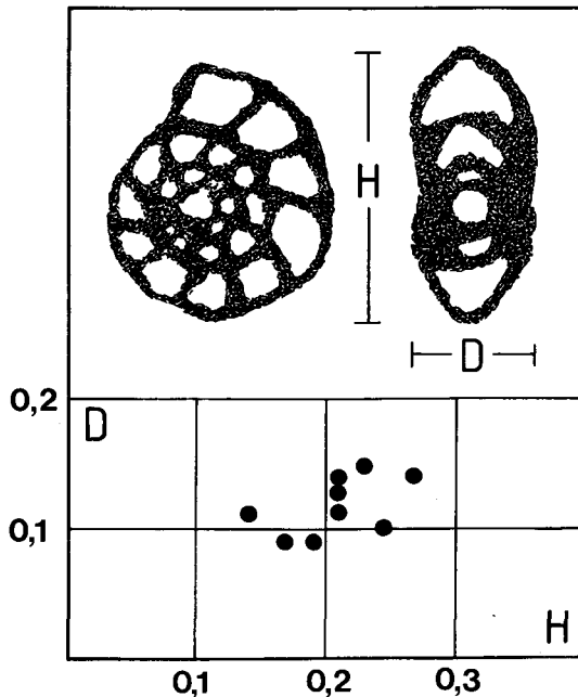
Abb. 5: Gehäusevariabilität von Montcharmontia apenninica (DE CASTRO) in den Rudistenkalken der Pletzachalm und des Stroblers Weißenbachtals. (Angaben in mm).
