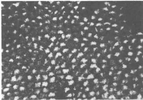
Fig. 3: Alveolites fecundus LECOMPTE, 1939 Querschliff mit alveolitiden Korallen- querschnitten TAB 2
