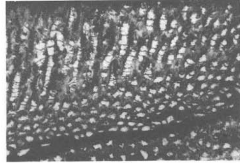
Fig. 4: Alveolites fecundus LECOMPTE, 1939 Längsschliff. Im unteren Bildbereich neuerliche (ontogenetisch juvenile) Anfangslage (Koralliten ohne Septaldor- nen!) nach Wachstumsunterbrechung. TAB 2
