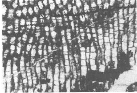
Fig. 2: Alveolites edwardsi LECOMPTE, 1939 Längsschliff TAB 4
