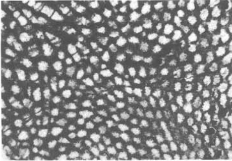
Fig. 1: Alveolites edwardsi LECOMPTE, 1939 Querschliff mit Koralliten in typisch alveolider Ausbildung. Deutlich erkennbare Septaldornen. TAB 4
