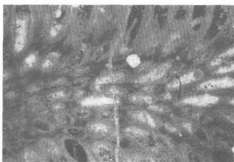
Fig. 4: Thamnopora reticulata (de BLAINVILLE, 1830) Längsschliff TAB 10
