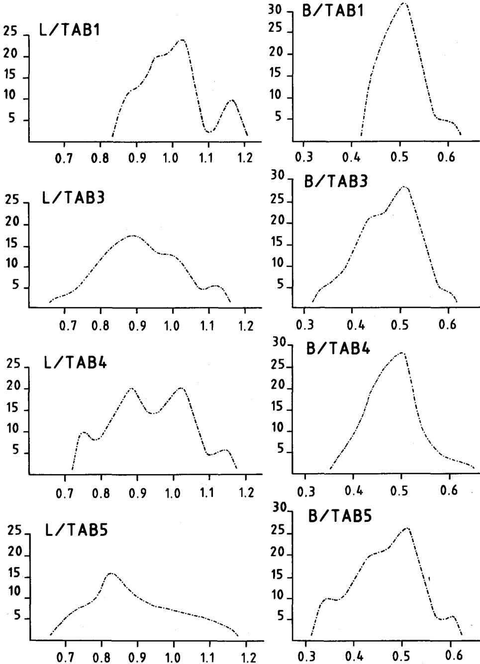
Abb. 3: Häufigkeitsverteilung langer (L) und kurzer (B) Korallitenquerschnittsachsen von Alveolites edwardsi (Korallenstöcke TAB 1, TAB 3, TAB 4, TAB 5). Abszisse: Maße in mm. Ordinate: Häufigkeit in %.
