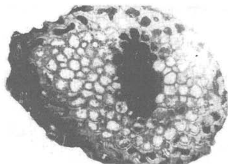
Fig. 1: Alveolites sp. Querschliff durch dendroid-ästige Kolonie. TAB 9
