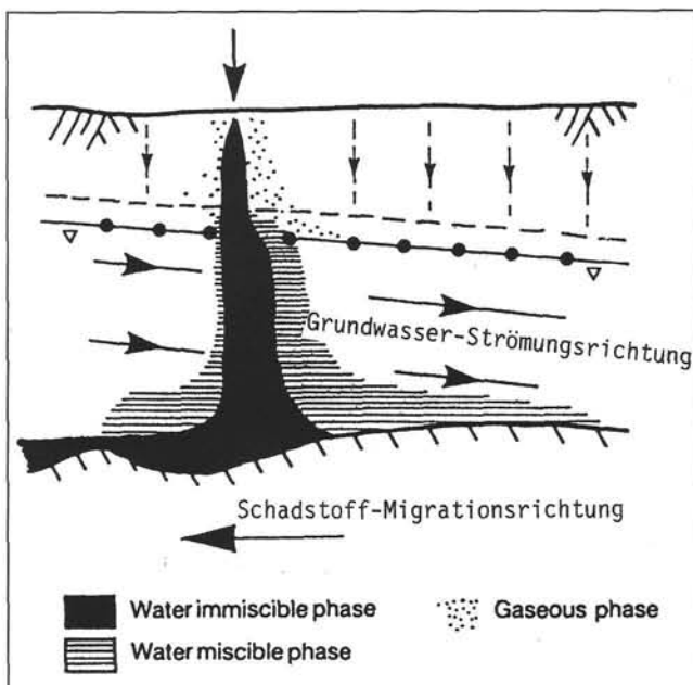
Abb. 1. Schadstoffversickerung und Migration von spezifisch schwereren Phasen trifft nicht entlang der Grundwasserspiegeloberfläche nach deren Einfallrichtung, sondern füllen das Relief des Grundwasserstauers und folgen dessen Abdachung. Ergänzt nach DOWNING & WILKINSON (1991).
