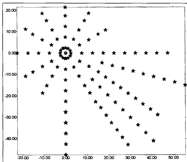
Abb. 4. Anordnung des modifizierten Meßrasters nach dem System der WENNER-Kartierung in Form eines Sternes mit der Option der Erweiterbarkeit im abstromigen Sektor. Prinzipiskizze ohne Maßstab mit zentraler Einspeiskünette oder Bohrung (Kreis mit Punkt) und Elektrodenmeßpunkten (Sterne).
