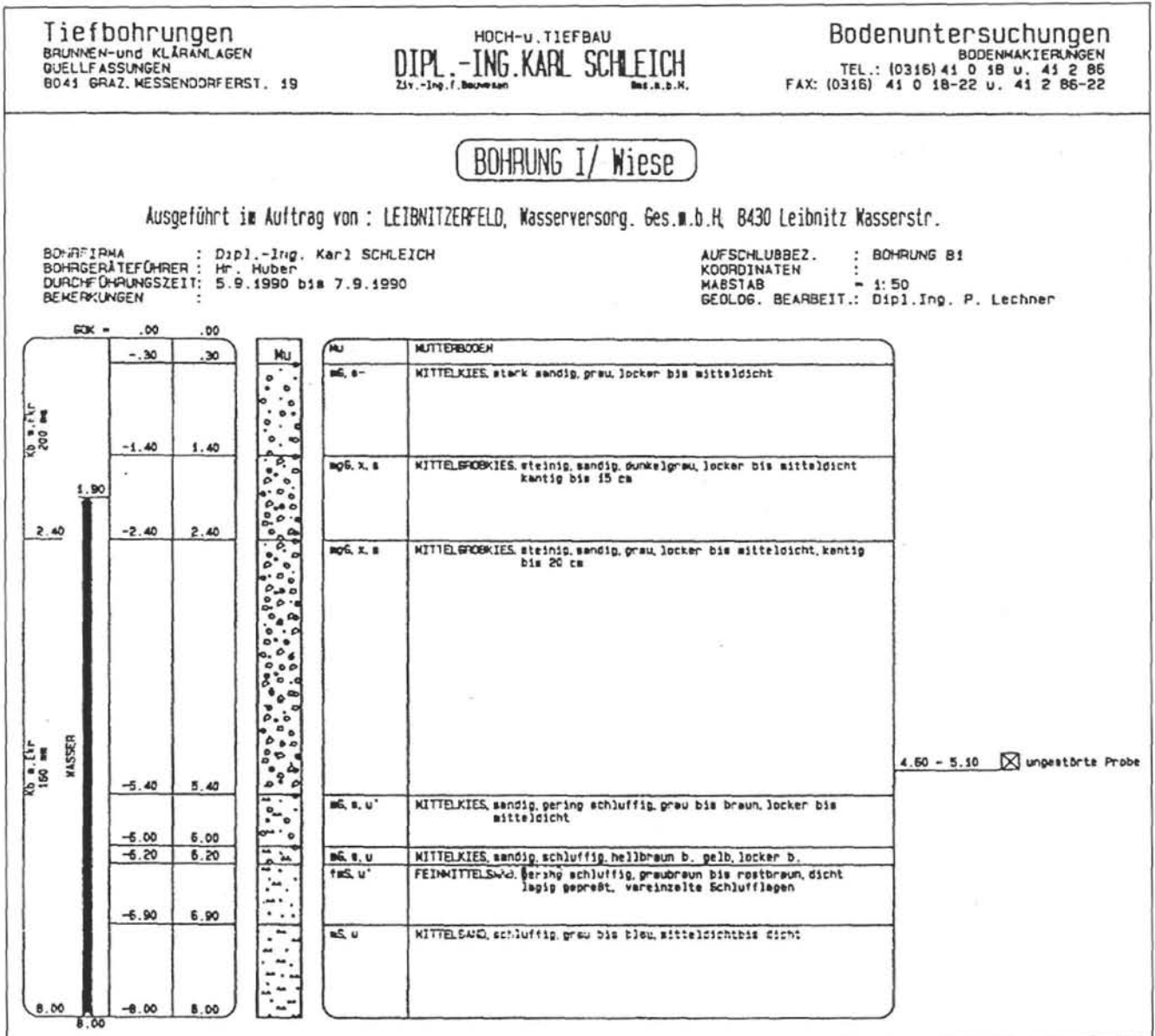
Abb. 6. Schichtenverzeichnis der Bohrung I (Aufschlußbohrung für den Bau des Notversorgungsbrunnens) im alluvialen Talboden der Haslacher Au.
