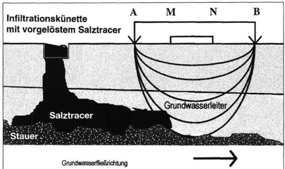
Abb. 2. Das Meßprinzip des geoelektrischen Nachweises künstlich eingespeister Salztracer. A – B: Außenelektroden (Stromeinspeisung I), M – N: Innenelektroden (Potentialmessung U).
