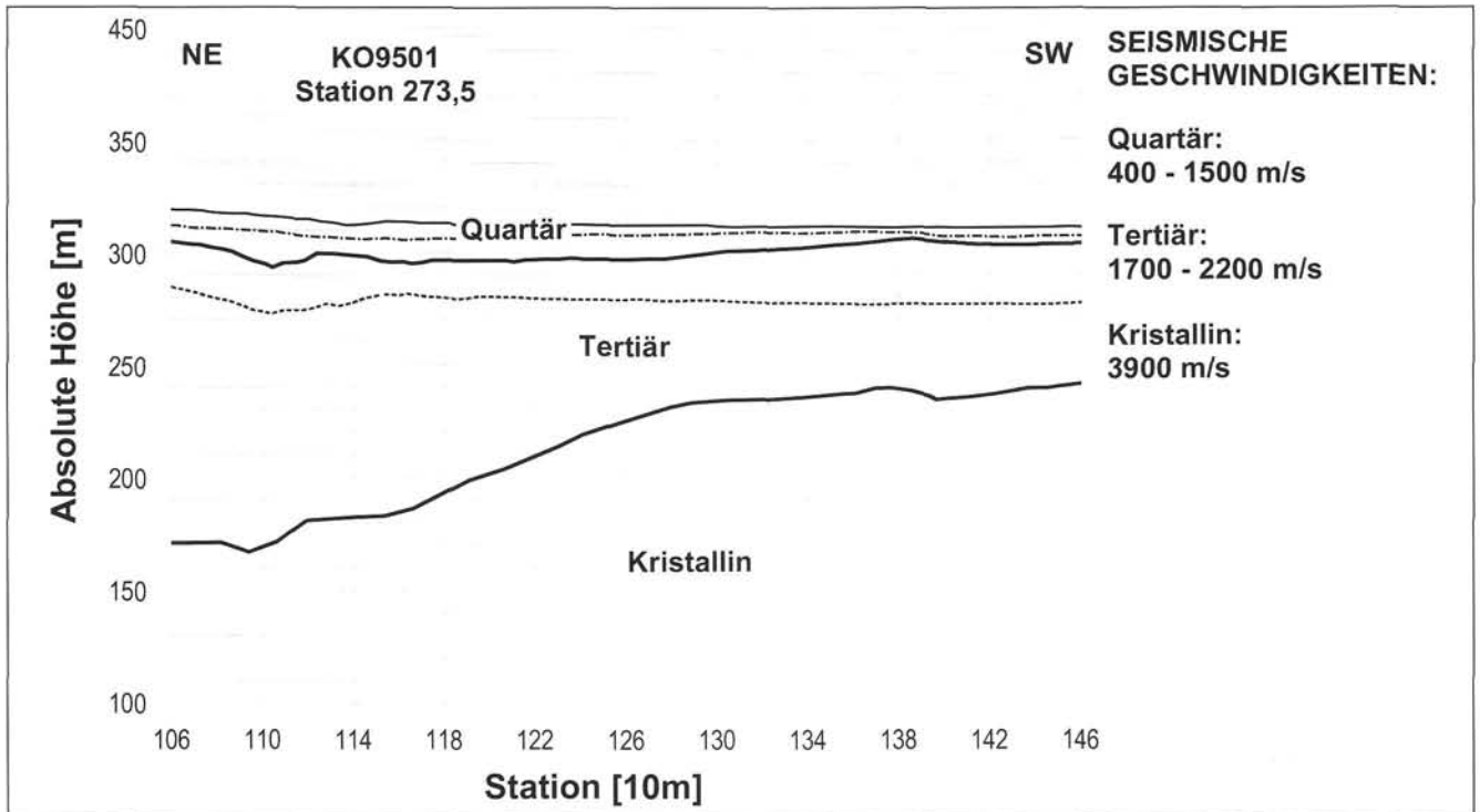
Abb. 4 Auswertung der Refraktionsseismik Profil KO9401, Geophonposition 106-146. Deutlich ist der treppenartige Anstieg des kristallinen Untergrundes (entlang von Brüchen?) im NE-Abschnitt des Profiles erkennbar. Die Unterteilungen im Quartär bzw. im Tertiär basieren auf seismischen Geschwindigkeitsunterschieden, können jedoch lithologisch nicht näher spezifiziert werden. Der Kreuzungspunkt mit Profil KO9501 bei Station 115,5.
