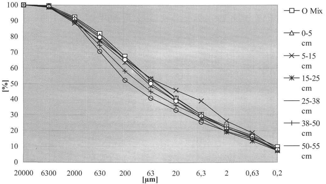
Abb. 8 Bereich der Kornsummenkurven der mineralischen Basisbarriere von Gmünd. O_{\text{Mix}} ist eine Oberflächenmischprobe. Der Anteil der Tonfraktion ( < 2 \mu\text{m} ) liegt im wesentlichen über 20%.
