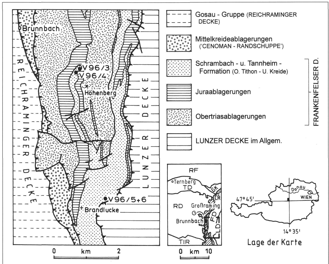
Abb. 1 Geologische Übersicht der Frankenfelder Decke im Bereich der Weyerer Bögen nach EGGER & FAUPL (1999). Tektonische Übersicht: RF – Rhenodanubische Flyschzone, GK – Grestener Klippenzone, TD – Ternberger Decke, RD – Reichraminger Decke, G – Gosau-Gruppe auf der Reichraminger Decke, TIR – Tirolikum, CR – „Cenoman-Randschuppe“, FD – Frankenfelder Decke, LD – Lunzer Decke.
