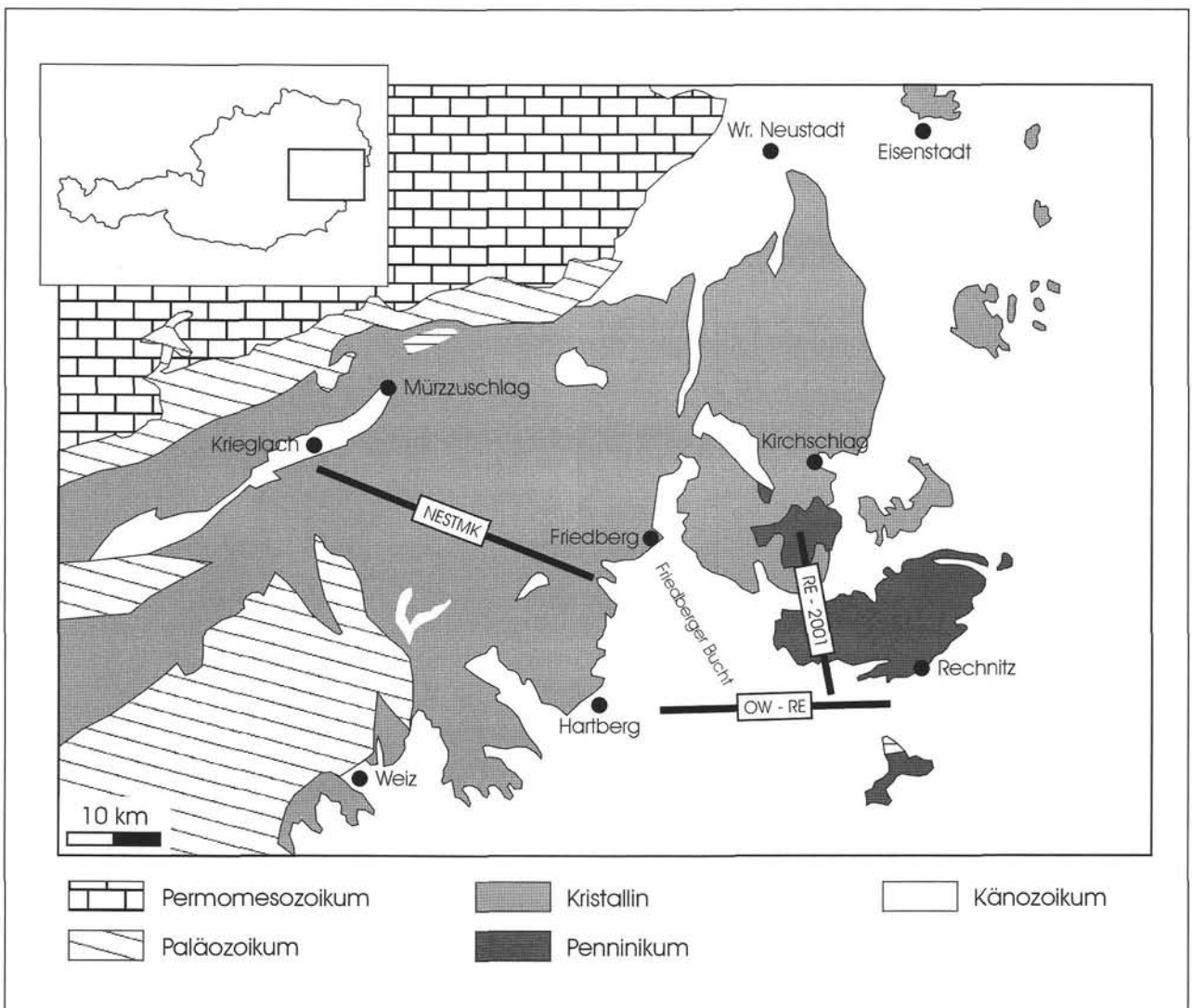
Abb. 1 Geologische Übersicht des Übergangsbereiches der Ostalpen zum Pannonischen Becken nach BECK-MANNAGETTA & BRAUMÜLLER (1986). Lage und Verlauf der tiefenreflexionsseismischen Profile Nordoststeiermark 1996 (NESTMK), Oberwart-Rechnitz 1992, 1993 und 1997 (OW-RE) und Rechnitz 2001 (RE-2001).
