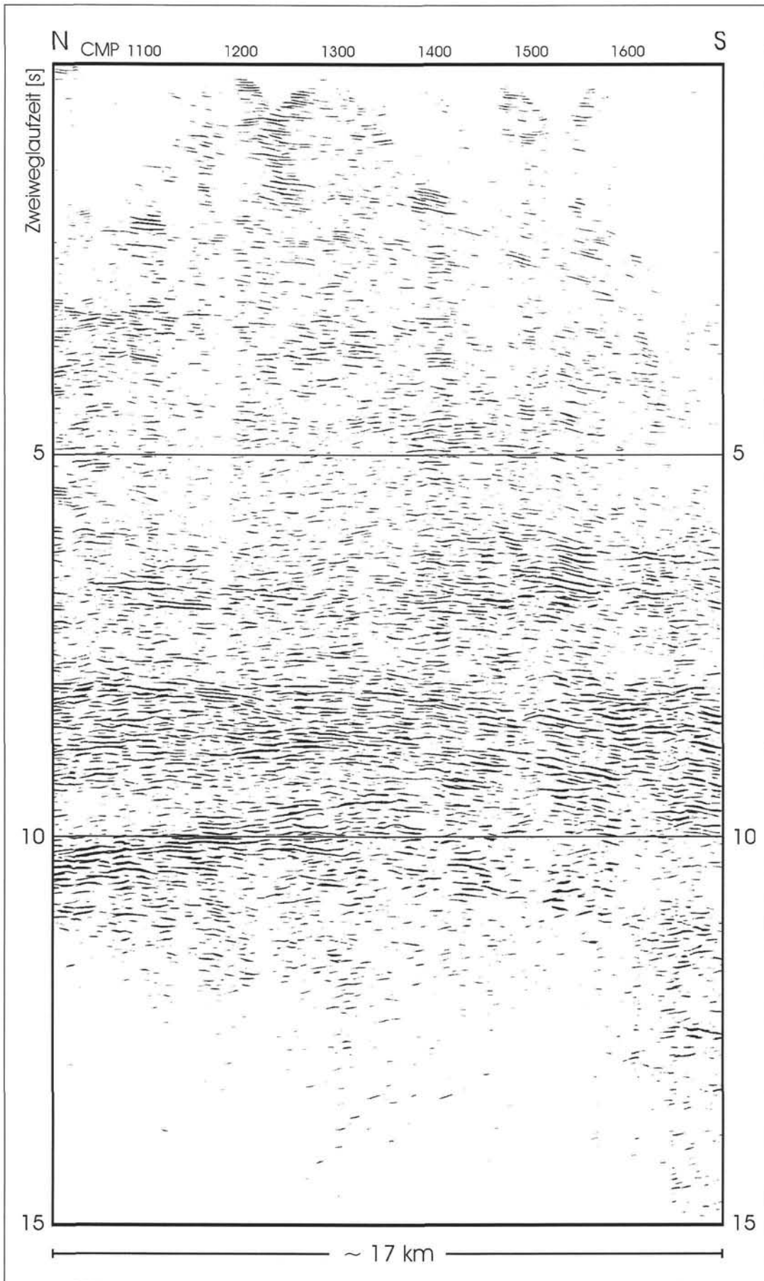
Abb. 2 „Stark“ kohärenzgefilterte und amplitudenmodifizierte ( Vernachlässigung von Amplituden kleiner 0,5) Stapelsektion (CMP 1007 bis 1697) bis zu einer Zweiweglaufzeit von 15 s ( dies entspricht unter der Annahme einer Geschwindigkeit von 6000 m/s einer Tiefe von 45 km). Bezugsniveau = Adria-Null, Darstellung horizontal gedehnt ( H : V = 150 : 100), Lage der CMP's siehe Abb. 3.
