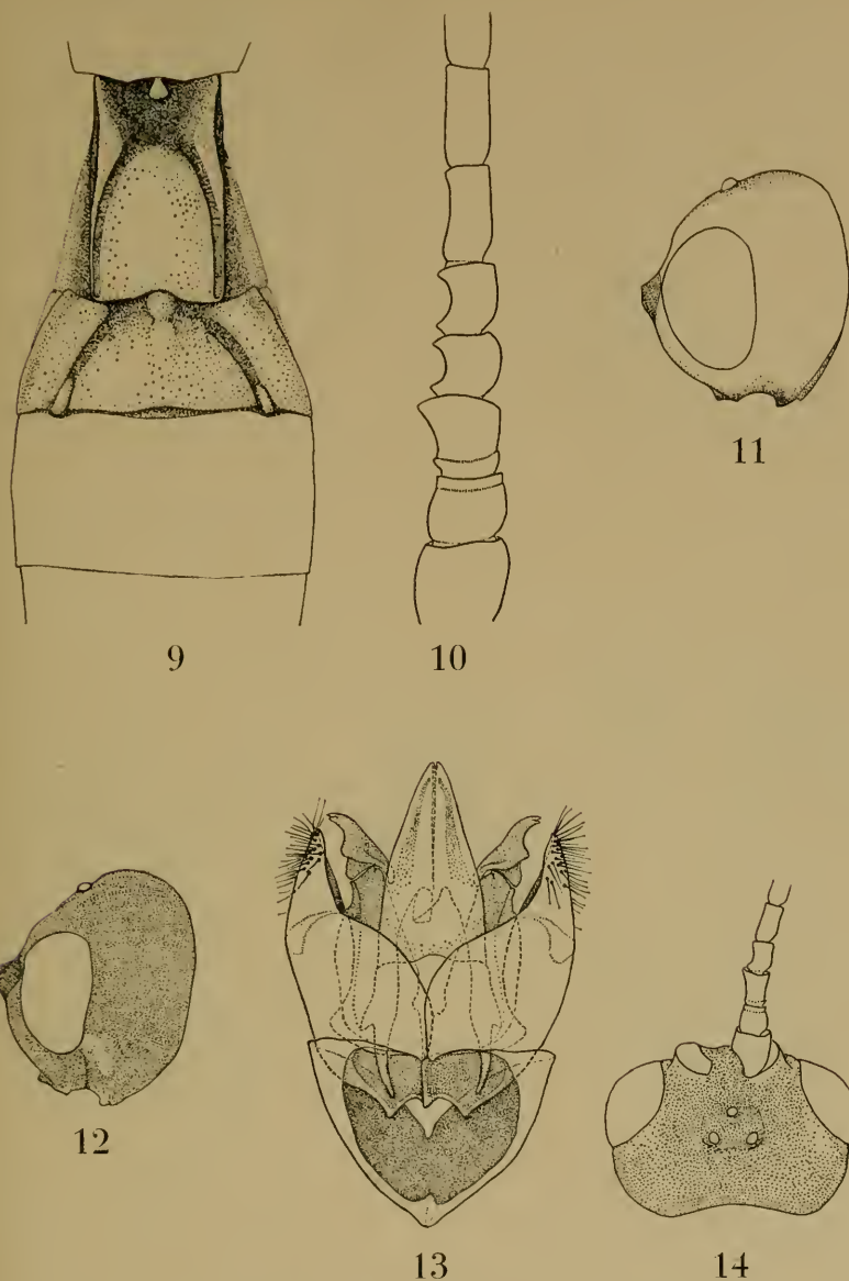
Abb. 9: Coeloides unguicularis watanabei ssp. n., ♂, Holotypus. Vordere Gastertergite.
