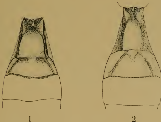
Abb. 1: Coeloides melanotus Wesm., ♀. Vordere Gastertergite.
