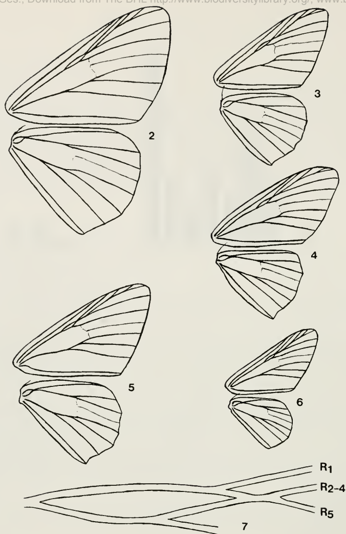
Abb. 2-7. 2-6: Flügelgeäder der Typusarten der Subgenera Glossotrophia (2: G. confinaria H.-S.), Libanonia (3: G. semitata PRT.), Bicalcarella (4: G. terminata WILTS.), Parenzaniella (5: G. asellaria H.-S.), Microglossotrophia (6: G. alfieri WILTS.). 7: Detail der Äderung (Vorderflügel-Areole) von Glossotrophia ( Microglossotrophia ) buraimana WILTS.
