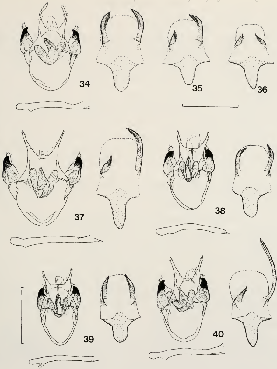
Abb. 34-40: 34: Glossotrophia (G.) mentzeri sp. n., Holotypus, ♂ Genitalapparat. 35: Glossotrophia (G.) mentzeri sp. n., Paratypus, 8. Sternit (f. antisoceras ). 36: Glossotrophia (G.) mentzeri sp. n., Paratypus, 8. Sternit (f. brevicerata ). 37: Glossotrophia (G.) alba africana subsp. n., Holotypus, ♂ Genitalapparat. 38: Glossotrophia (G.) rufomixtaria subsp. n.? (Marokko), ♂ Genitalapparat. 39: Glossotrophia (G.) rufomixtaria saharensis subsp. n., Holotypus, ♂ Genitalapparat. 40: Glossotrophia (G.) diffinaria PRT. (S.-Griechenland), ♂ Genitalapparat. (Skala der Abb. 34-40 = 1 mm).
