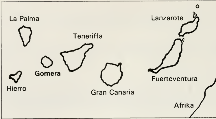
Abb. 12: Lage der Insel Gomera im kanarischen Archipel.
