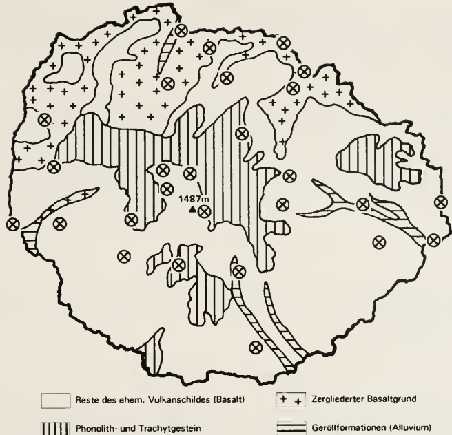
Abb. 14: Gomera, Verbreitung der bekannten Zikadenarten in bezug auf die geologische Gliederung der Insel (nach MITCHELL-THOMÉ 1976, verändert).
