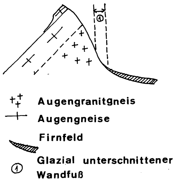
Abb. 2: Schematisches NE—SW Querprofil durch die Hohe Leier (2774 m).
