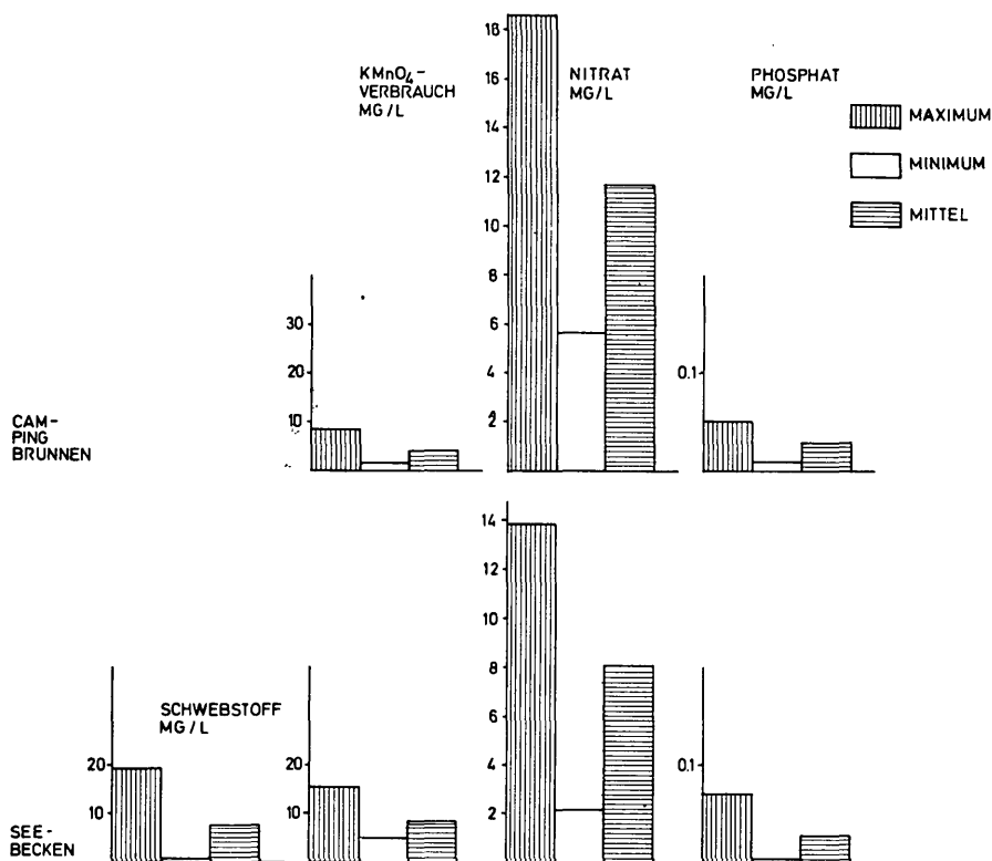
Abb. 4: Röcksee-Schwankungsbreiten des Schwebstoffgehaltes, des KMnO 4 -Verbrauchs sowie des Nitrat- und Phosphatgehaltes.
