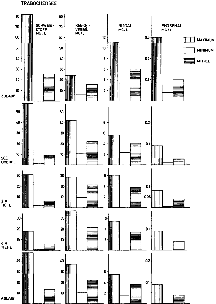
Abb. 1: Trabochersee-Schwankungsbreiten des Schwebstoffgehaltes, des KMnO 4 -Verbrauchs sowie des Nitrat- und Phosphatgehaltes.
