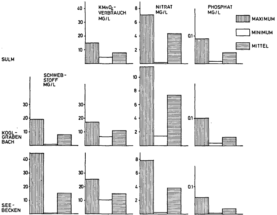
Abb. 2: Sulfsee-Schwankungsbreiten des Schwebstoffgehaltes, des \text{KMnO}_4 -Verbrauchs sowie des Nitrat- und Phosphatgehaltes.
