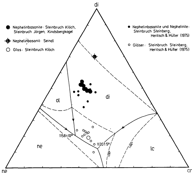
Abb. 1: Im Diagramm Diopsid-Nephelin-Sanidin nach SOOD, PLATT & EDGAR 1970 liegen die basaltischen Gesteine des Steinberges bei Feldbach und die Nephelinbasanite des Klöcher Vulkangebotes eng beisammen, nur das offenbar sekundär stärker veränderte Gestein vom Seindl liegt abseits. In beiden Vulkangebieten entstehen weitgehend gleichartige basaltische Gläser durch Abkühlung von restlichen Schmelzen, die durch Ausscheidung von Diopsid an die Phasengrenze Diopsid — Nephelin gelangen.
