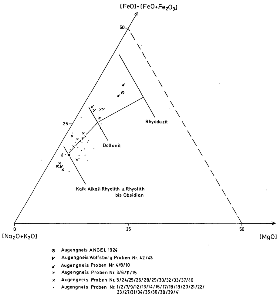
Abb. 5: Die 41 Augengneisproben des Augengneiszuges Hochalpe–Gleinalpe–Stubalpe, der Augengneis nach ANGEL 1924 sowie die 2 Augengneise von Wolfsberg im Variationsdiagramm [\text{FeO}] - [\text{Na}_2\text{O} + \text{K}_2\text{O}] - [\text{MgO}] nach NOCKOLDS & ALLEN 1954. Zum Vergleich sind ferner die Mittelwerte für Rhyodazit – Dellenit – Kalkalkali Rhyolith und Rhyolith bis Obsidian nach NOCKOLDS 1954, siehe Text, eingetragen. Die Signaturen sind so ausgewählt, daß sie mit der Tab. 4 und 5 im Einklang stehen.
