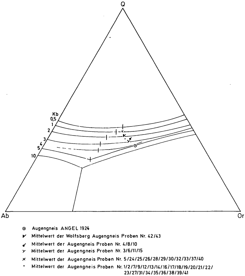
Abb. 7: Die Mittelwerte der nach steigenden \text{SiO}_2 -Werten gemittelten Augengneisproben der Hochalpe–Gleinalpe–Stubalpe, der Augengneis nach ANGEL 1924 sowie der Mittelwert der 2 Augengneisproben von Wolfsberg sind im Diagramm Q–Ab–Or nach LUTH et al. 1964, siehe Text, eingetragen.
