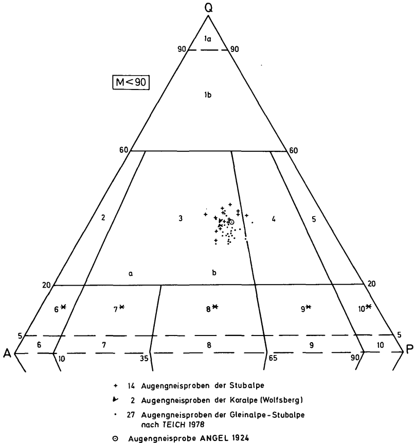
Abb. 2: Die Augengneisproben des Augengneiszuges der zentralen und südlichen Stubalpe im Diagramm Q–A–P nach STRECKEISEN 1973 für Plutonite. Zum Vergleich sind der Augengneis nach ANGEL 1924, die 27 Augengneisproben der Hochalpe–Gleinalpe–nördliche Stubalpe nach TEICH 1978 sowie die Augengneise von Wolfsberg, siehe Text, eingetragen.
