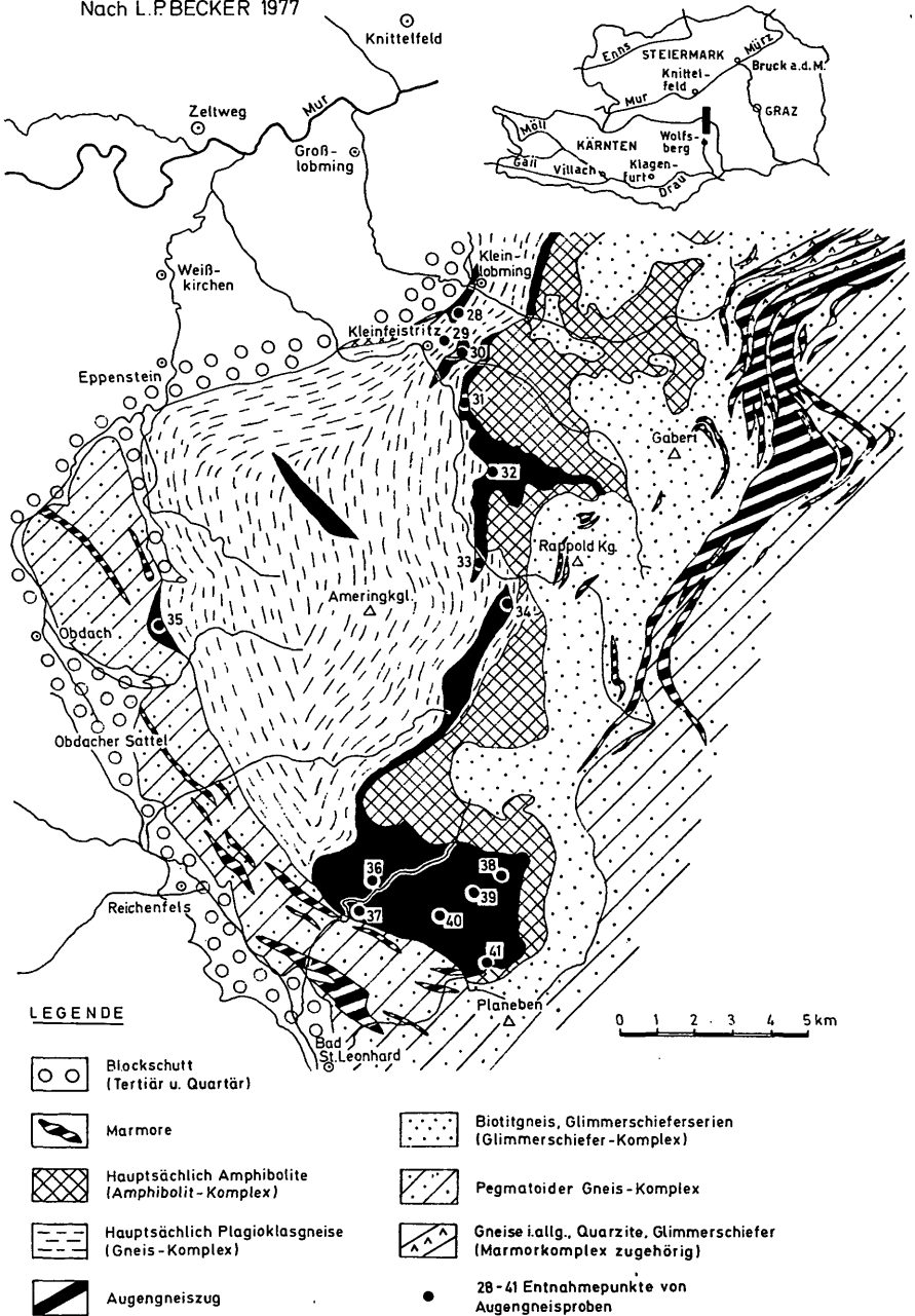
Abb. 1: Geologische Übersichtskarte des Stubalpenzuges nach BECKER 1977. Die Entnahmepunkte von 14 Augengneisproben aus dem Augengneiszug der zentralen und südlichen Stubalpe sind mit Nummern in die geologische Übersichtskarte eingetragen. Die Nummern sind dieselben wie in Tab. 1.
