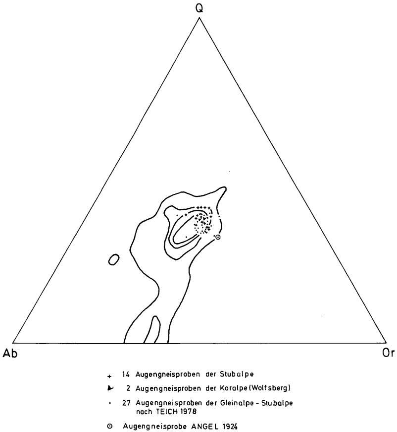
Abb. 3: Die Augengneisproben des Augengneiszuges der zentralen und südlichen Stubalpe im Diagramm Q-Ab-Or für Vulkanite nach TUTTLE & BOWEN 1958. Zum Vergleich sind der Augengneis nach ANGEL 1924, die 27 Augengneisproben der Hochalpe-Gleinalpe-nördliche Stubalpe nach TEICH 1978 sowie die Augengneise von Wolfsberg, siehe Text, eingetragen.
