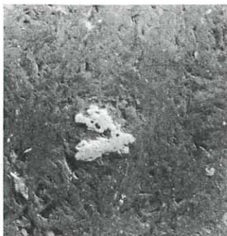
Abb. 3: Rasterelektronenmikroskopische Aufnahme eines Ilmenit-Kornes in heller Lage des Tuffits vom Rechberg bei Frohnleiten, Steiermark. Das hellgraue, lappig und löchrig ausgebildete Ilmenit-Korn hat einen Durchmesser von 0,03 mm; dunkelgrau: silikatische Mineralien.
