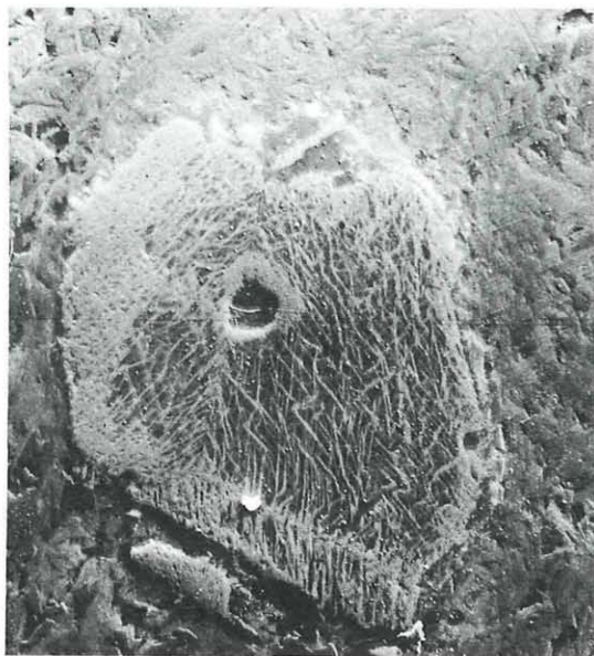
Abb. 4: Rasterelektronenmikroskopische Aufnahme eines zu tafeligen Anatasaggregaten umgewandelten Ilmenit-Kornes aus heller Lage des Tuffits vom Rechberg bei Frohnleiten, Steiermark. Andeutungen von Kristallflächen sind zu beobachten. Durchmesser des pseudomorphisierten Kornes 0,15 mm.
