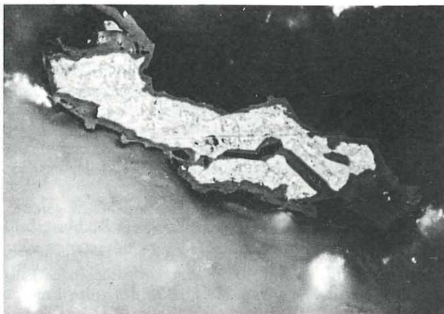
Abb. 5: Erzmikroskopische Aufnahme (Öl) eines unregelmäßigen Magnetit-Kornes, das sekundär randlich in Eisenhydroxid umgewandelt ist, aus heller Lage des Tuffits vom Rechberg bei Frohnleiten, Steiermark. Größter Durchmesser des Magnetit-Kornes 0,09 mm.
