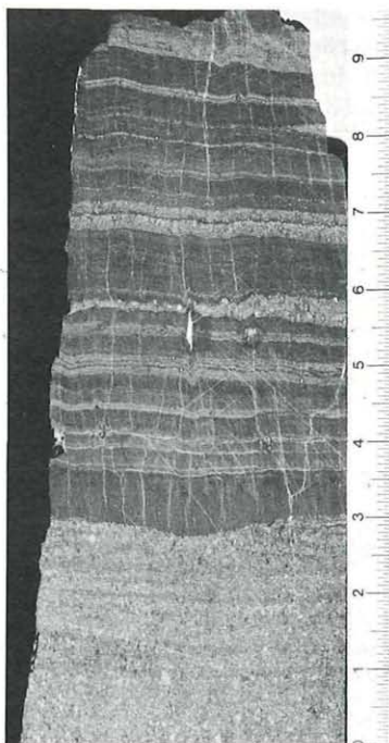
Abb. 2: Feingeschichteter Tuffit vom Rechberg bei Frohnleiten, Steiermark. Die hellen Lagen sind reich an Albit und führen vorwiegend spilitisches Material (Mineralbestand in Tab. 2), die dunklen Lagen haben die Zusammensetzung eines Tones mit Ilmeniteinstreuung (Mineralbestand in Tab. 2). Das gesamte Gestein ist leicht metamorph.
