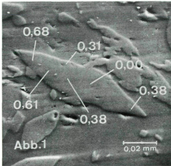
Abb. 1: Rasterelektronenmikroskopische Aufnahme des Querschnittes eines Na-Amphibol-(Crossit)-Stengels vom Fundpunkt Glasbachgraben bei Schlaining, Burgenland. Der Kern ist praktisch chromfrei. Gegen den Rand nimmt der Chromgehalt zu. Die Werte für \text{Cr}_2\text{O}_3 sind aus dem bekannten Eisengehalt des Crossites (HERITSCH 1965) von Dr. P. GOLOB mit Hilfe von Elektronenstrahlmikroanalysen bestimmt. Da bis zur Nachweisgrenze (etwa 2-3 \mu ) keine Einschlüsse beobachtet werden können, ist anzunehmen, daß das Chrom im Gitter des Na-Amphibols eingebaut ist.
