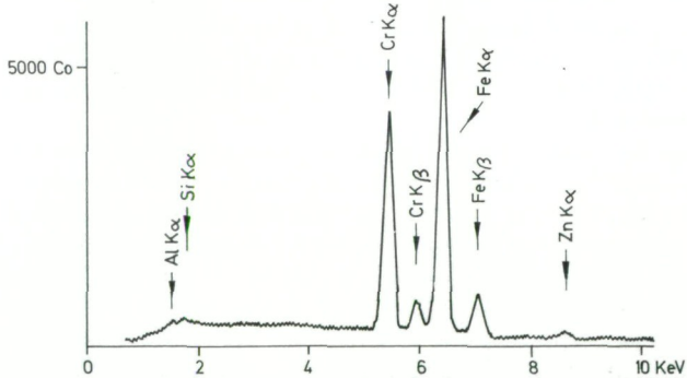
Abb. 2b und Abb. 2c: Elektronenstrahlmikroanalysen an den in Abb. 2a angegebenen Stellen. An diesem Korn ist fast keine Zonarität festzustellen. Die hauptsächlichen Elemente Cr und Fe gestatten es, einen Mischkristall mit 0,48 Chromit und 0,52 Magnetit zu berechnen, wobei die sehr geringen Anteile von Zn bzw. Al und Si unberücksichtigt bleiben.
