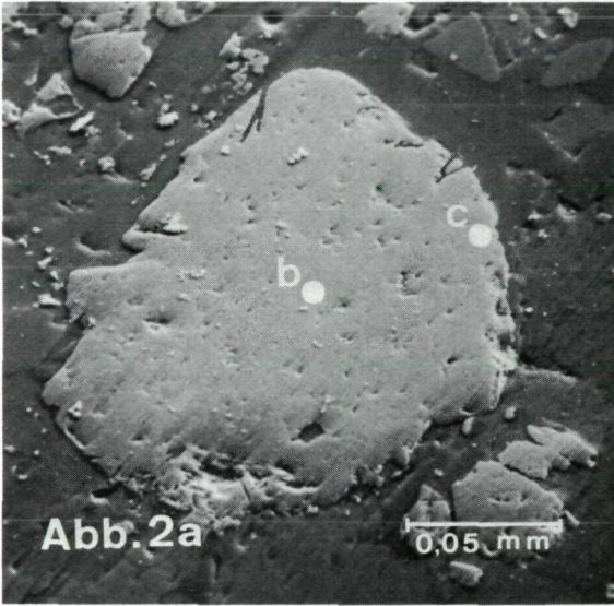
Abb. 2a: Rasterelektronenmikroskopische Aufnahme eines Mischkristalles von Chromit und Magnetit vom Fundpunkt Glasbachgraben bei Schlaining, Burgenland. Bis zur Nachweisgrenze mit Hilfe der Elektronenstrahlmikroanalyse ist nur eine einheitliche Phase festzustellen.
