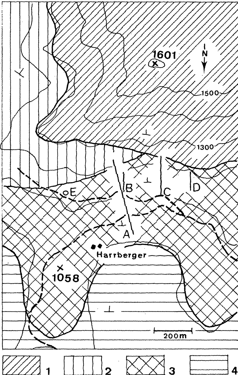
Abb. 1: Geologische Übersichtskarte und Lage der Profile am Nordabfall des Hochlantschstocks im Bereich Harrberger.
